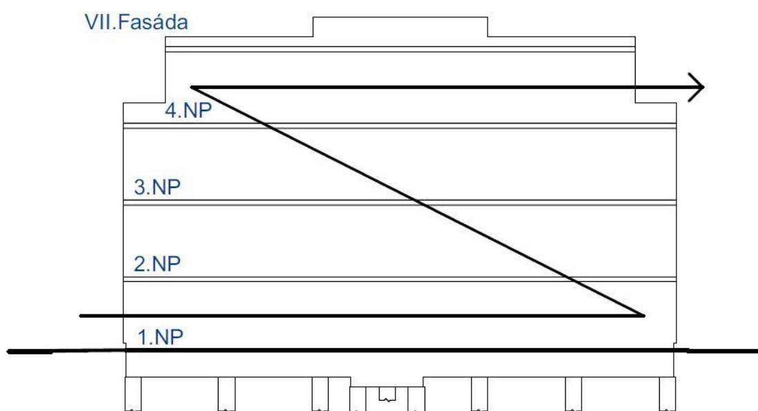
Obr. č.9 – Směr postupu výstavby pro etapy V a VI
