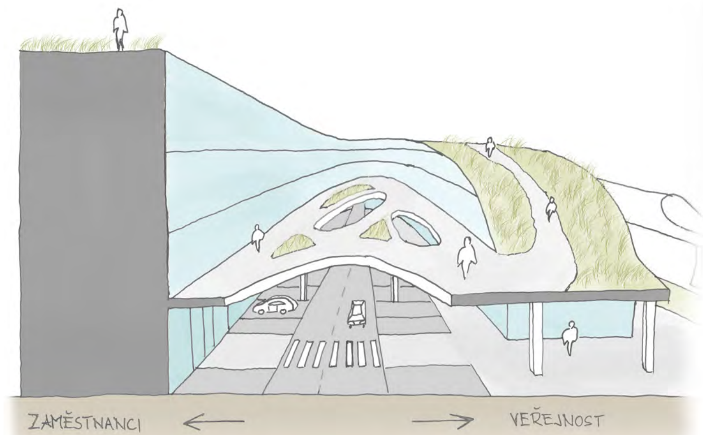
Řez administrativní budovou na hranici závodu Škoda
