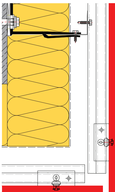
VNĚJŠÍ ROH A106
