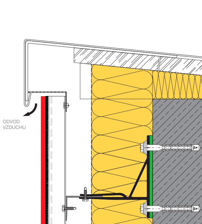
STŘEŠNÍ NAPOJENÍ - ATIKA A109
