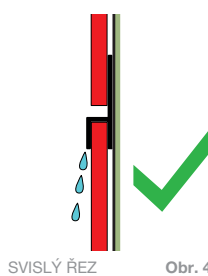
SVISLÝ ŘEZ
