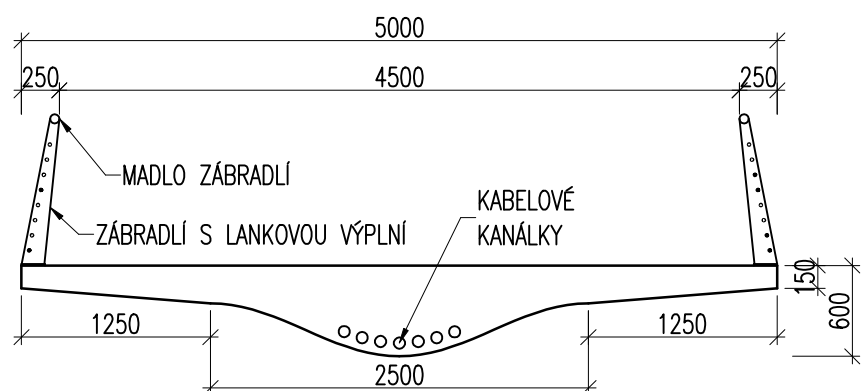
ŘEZ B-B M1:50
