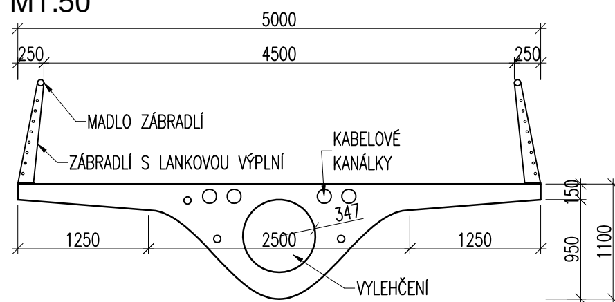
ŘEZ 3-3 M1:50
