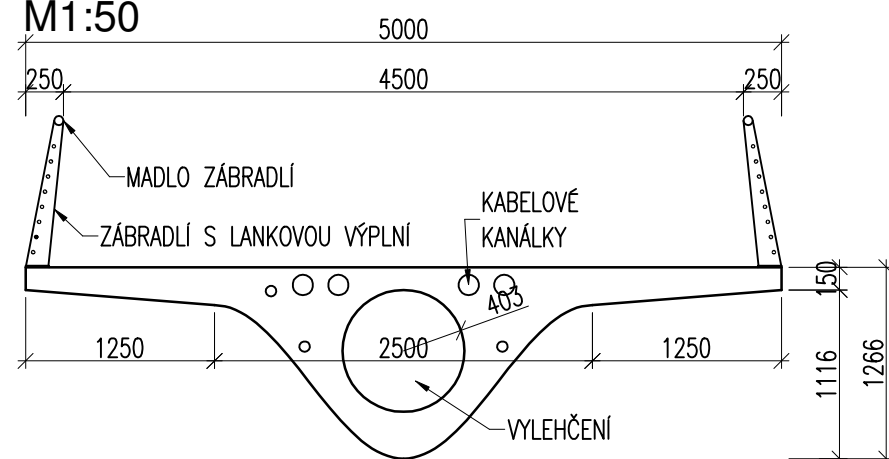
ŘEZ 2-2 M1:50
