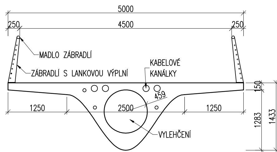
ŘEZ 1-1 M1:50
