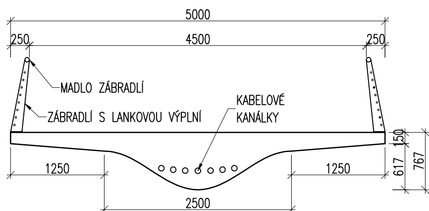
ŘEZ 4-4 M1:50
