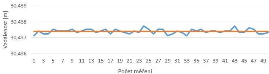
Horizontální natočení 20 gradů ~ 30 metrů
