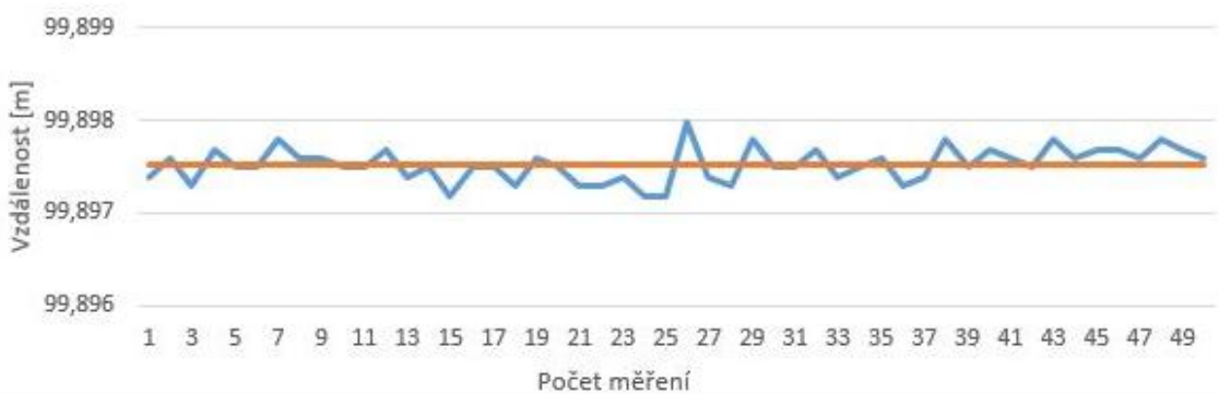
Vertikální natočení 60 gradů ~ 100 metrů- Leica
