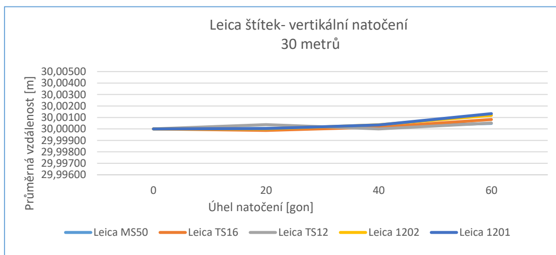
Obr. 29-Leica štítek ve vertikálním natočení- 30 metrů
