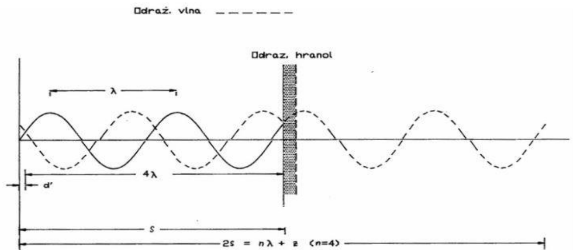
Obr. 1- Princip elektronického měření délek elektronickým dálkoměrem[1]
