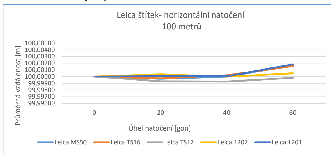
Obr. 28-Leica štítek v horizontálním natočení- 100 metrů
