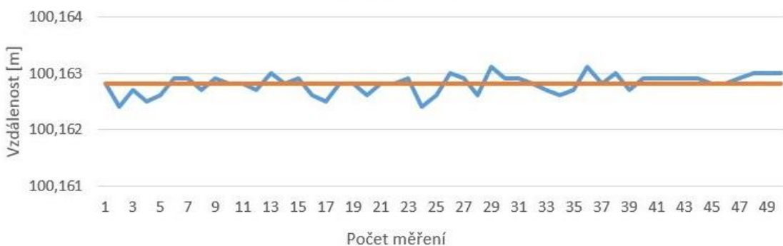
Horizontální natočení 60 gradů ~ 100 metrů- Leica
