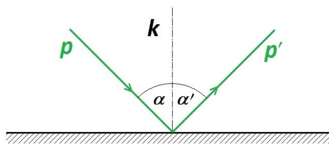
Obr. 3- Zákon odrazu [7]
