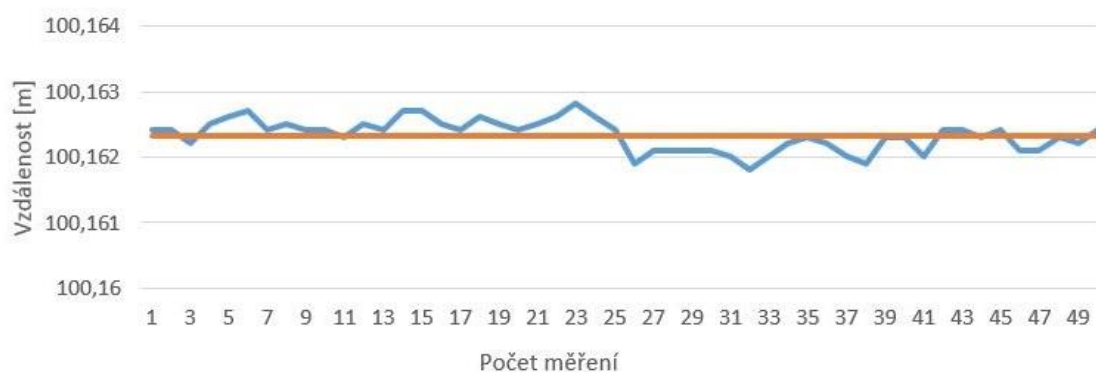
Horizontální natočení 40 gradů ~ 100 metrů- Leica
