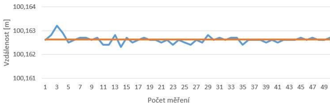
Horizontální natočení 20 gradů ~ 100 metrů- Leica
