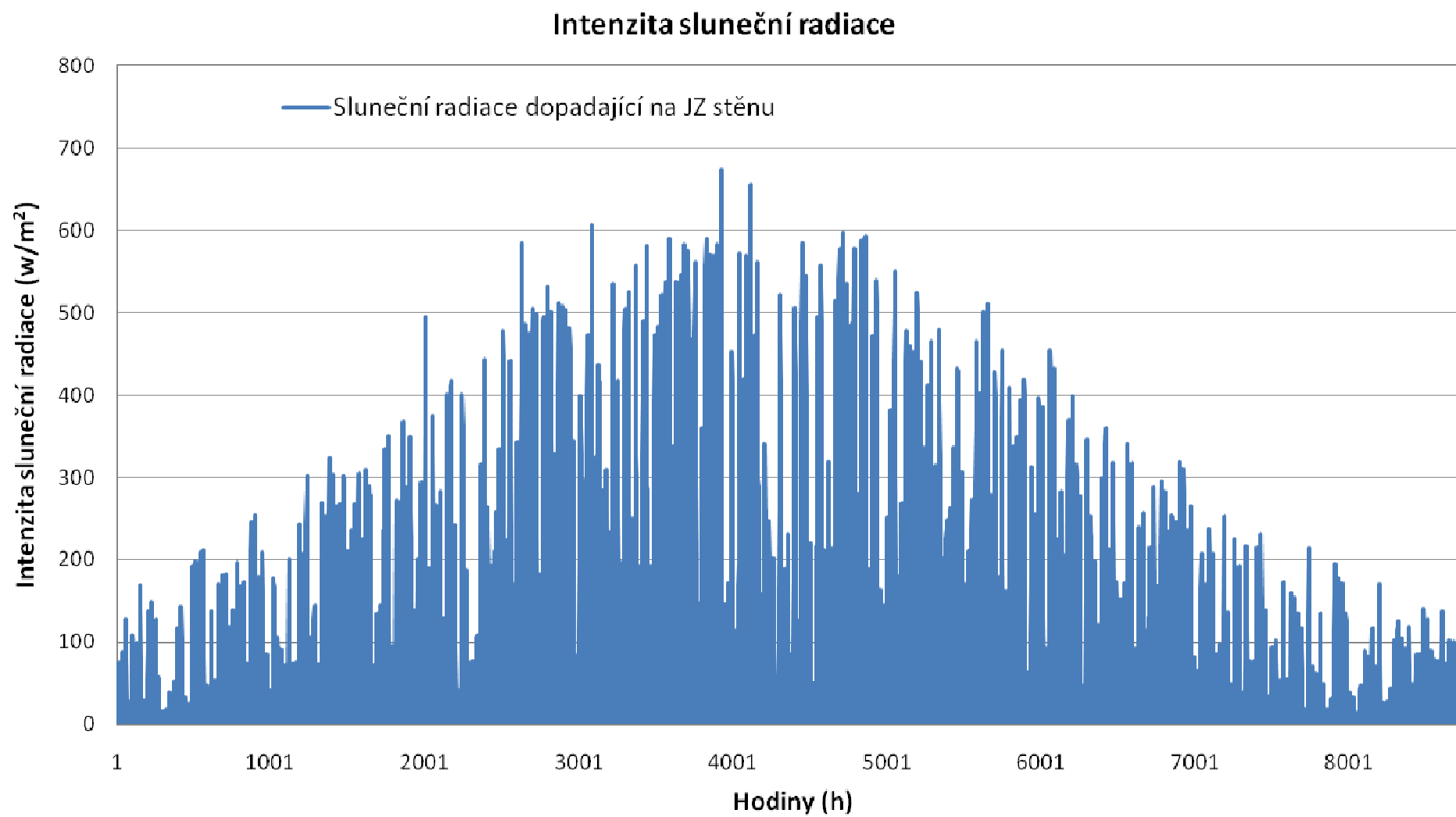
Příloha 3 Průběh intenzity sluneční radiace dopadající na JZ stěnu
