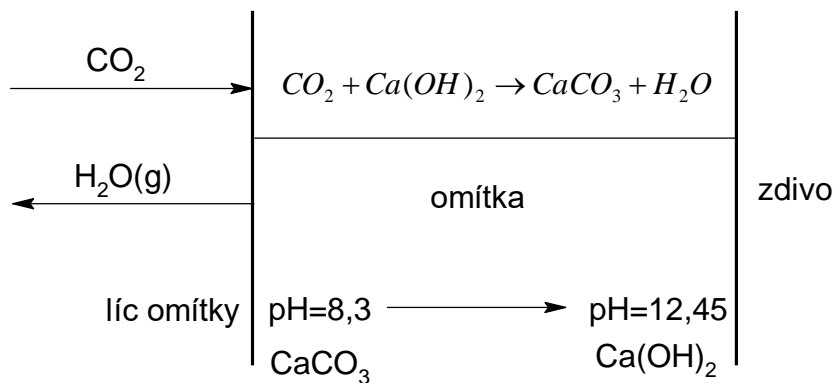
Obr. 4: Průběh karbonatace vápenné omítky [13]
