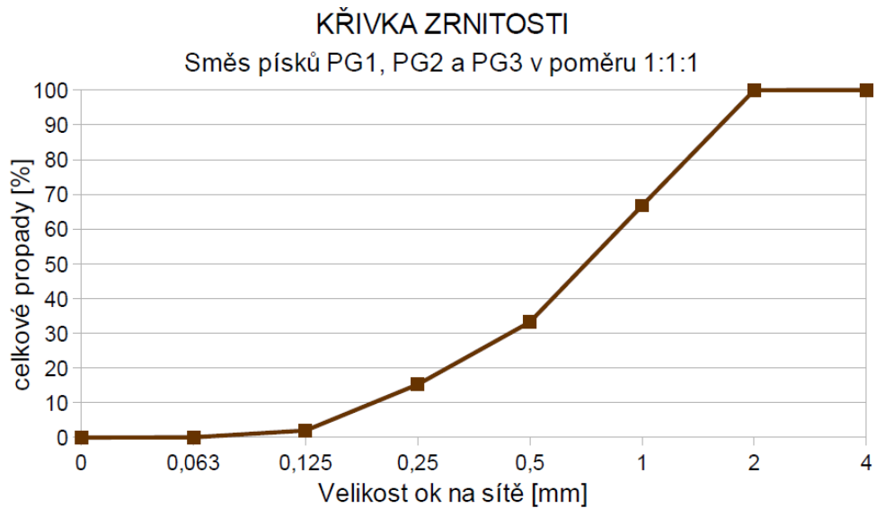
Obr. 43: Křivka zrnitosti směsi písků PG 1, PG 2 a PG 3 v poměru 1 : 1 : 1
