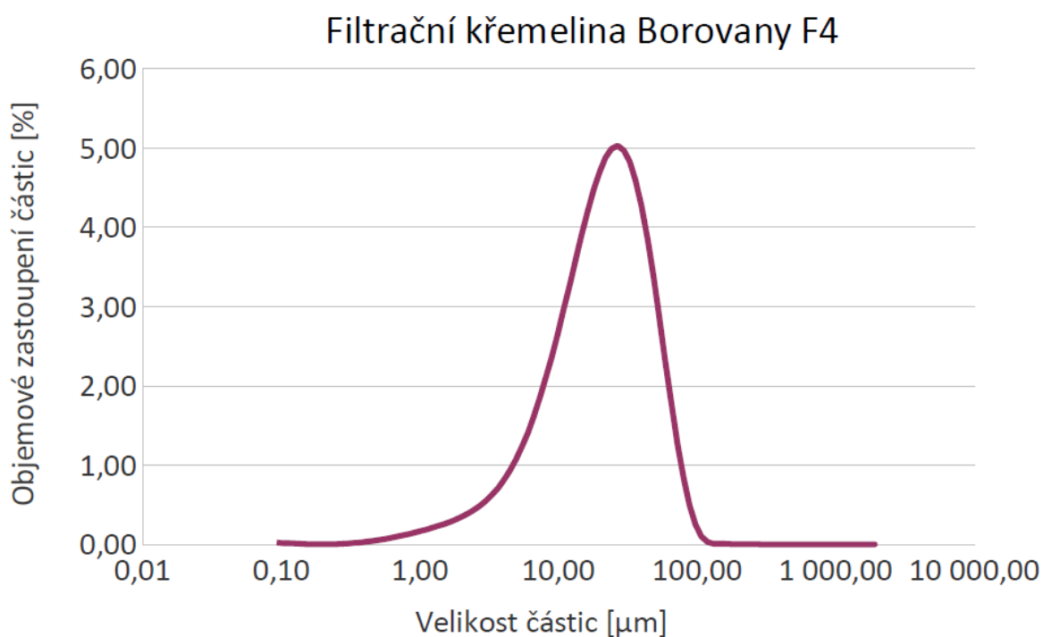
Obr. 40: Graf objemového zastoupení velikosti částic pro filtrační křemelinu F4 Borovany
