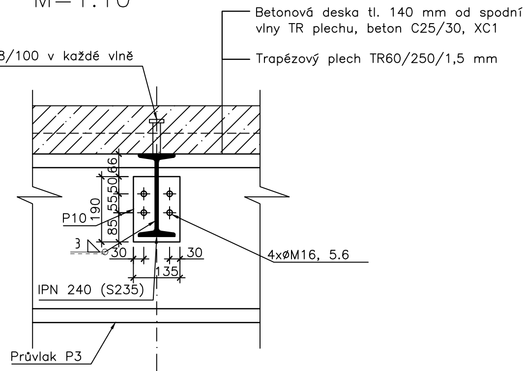
ŘEZ A-A: M=1:10
