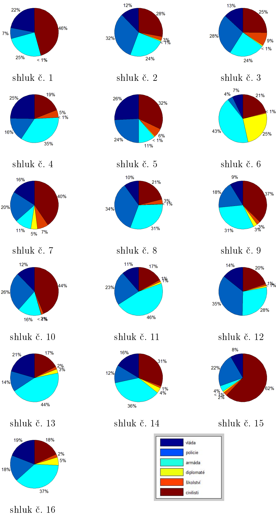
Obrázek 8: Cíle útoků [1]
