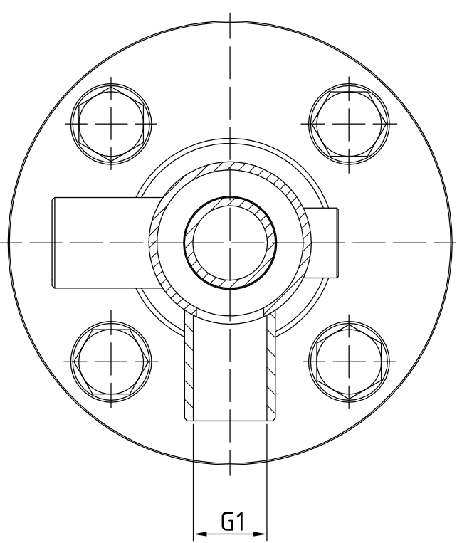
ŘEZ A-A MĚŘÍTKO 1 : 1
