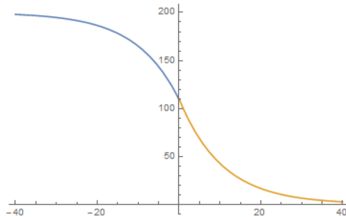
Obrázek 4.2: Funkce urgentnosti pro úkol s termínem
