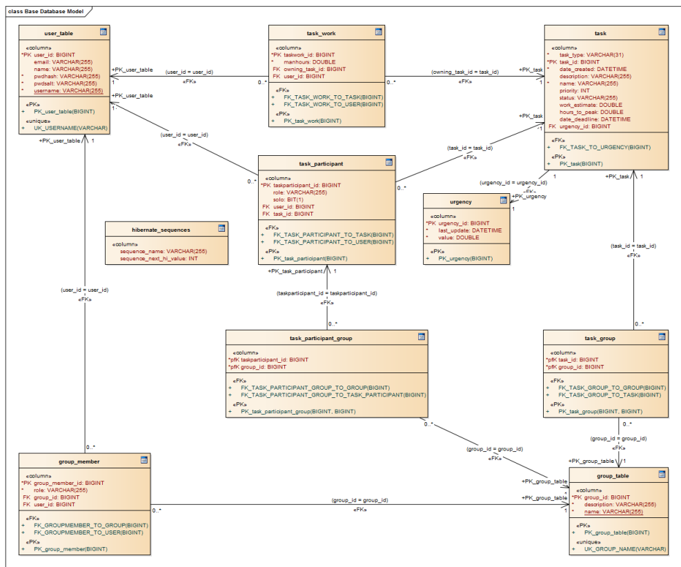
Obrázek G.1: Relační databázový model entit aplikace, vyjma nabídek
