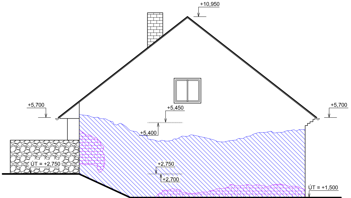
P-19: POHLED NA FASÁDU OD SEVEROZÁPADU:
