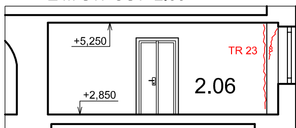
P-17: VNITŘNÍ POHLED PŘÍČKU Z MÍSTNOSTI 2.06
