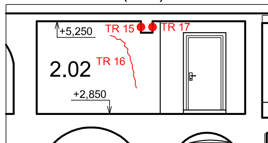
P-16: VNITŘNÍ POHLED NA JZ STĚNU LOŽNICE (2.02)
