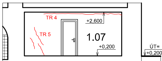
P-10: VNITŘNÍ POHLED NA PŘÍČKU Z POKOJE 1.07
