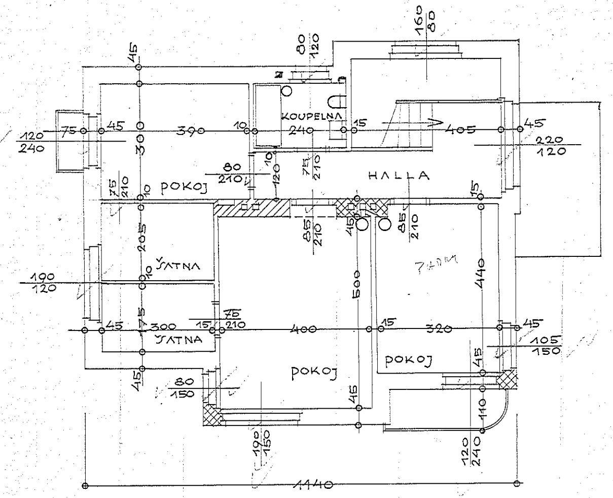
I PATRO,
