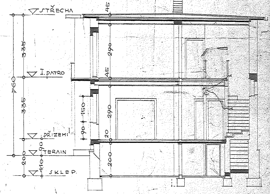
ŘEZ A-B,
