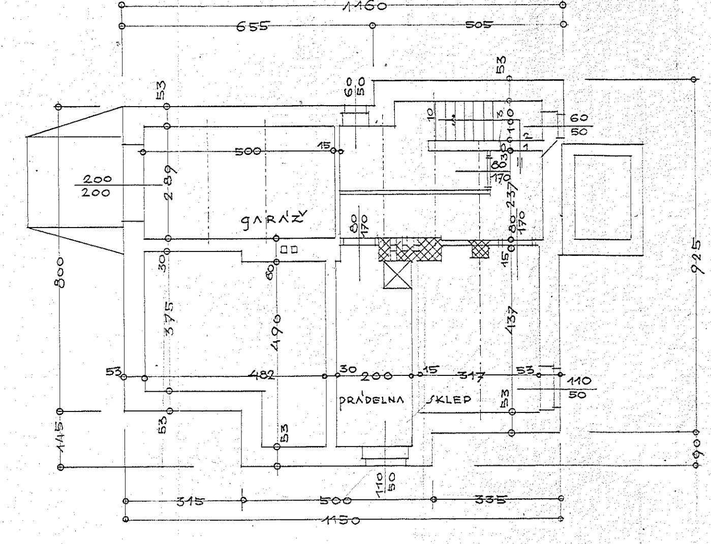
SKLEPY,
