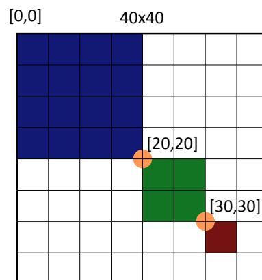
Obrázek 3.4: Příklad transformace
