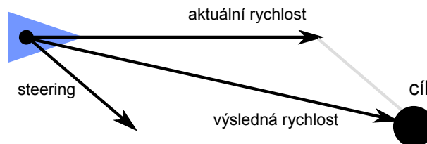
Obrázek 6.2: Seek
