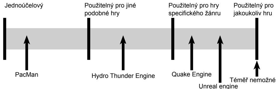
Obrázek 1.7: Modularita enginů
