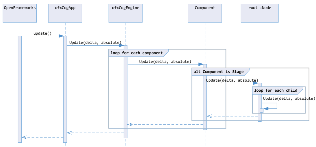
Obrázek 2.5: Aktualizace enginu
