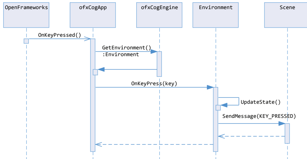
Obrázek 4.2: Zpracování událostí
