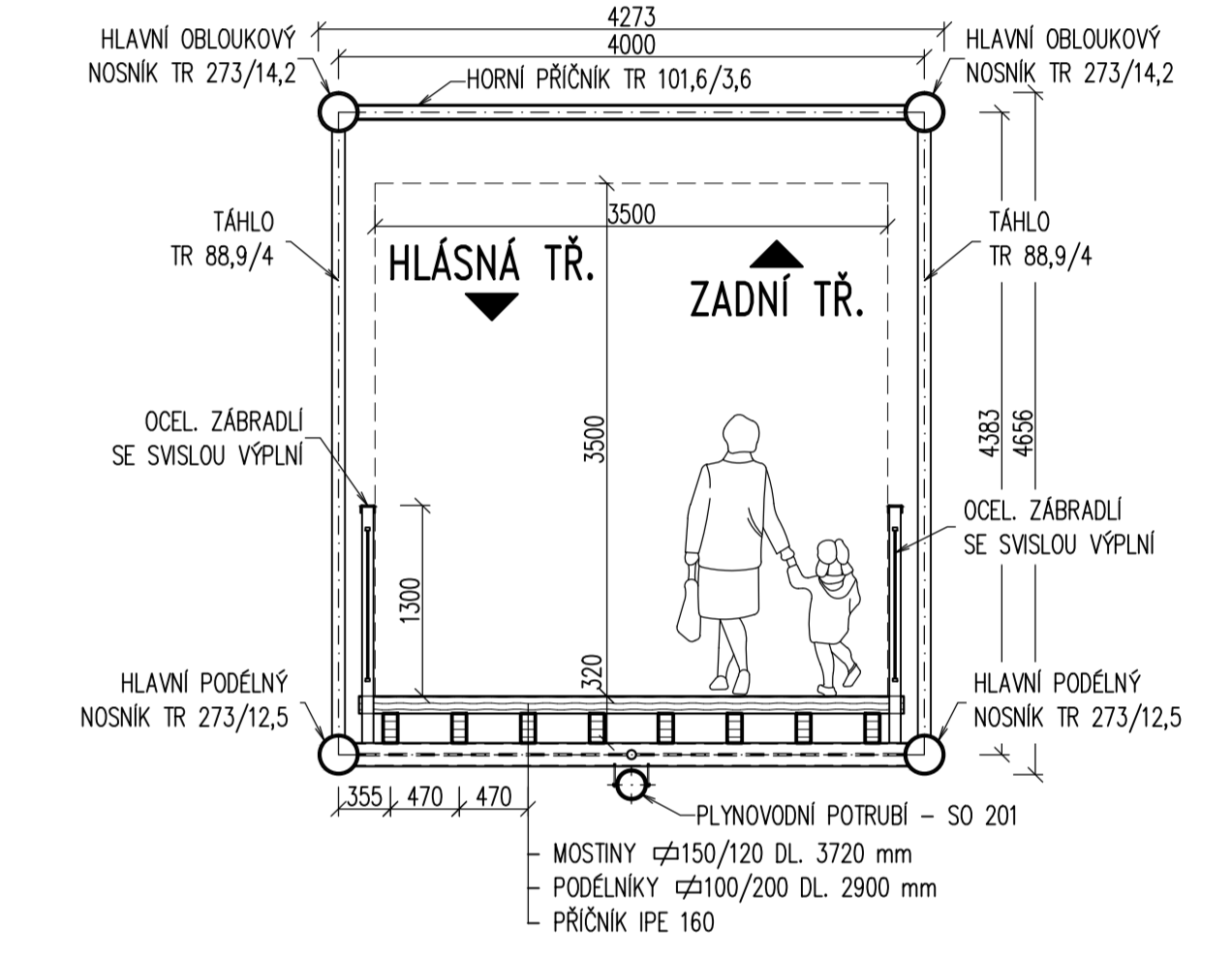
PRÍČNÝ ŘEZ A 1:50
