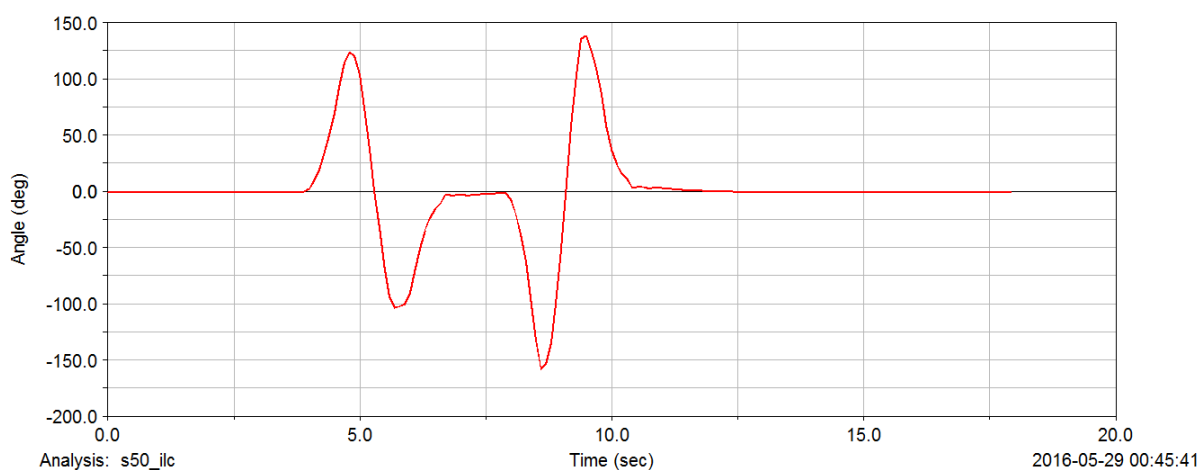
Př. 4 Úhel natočení volantu při simulaci v 50 km/h
