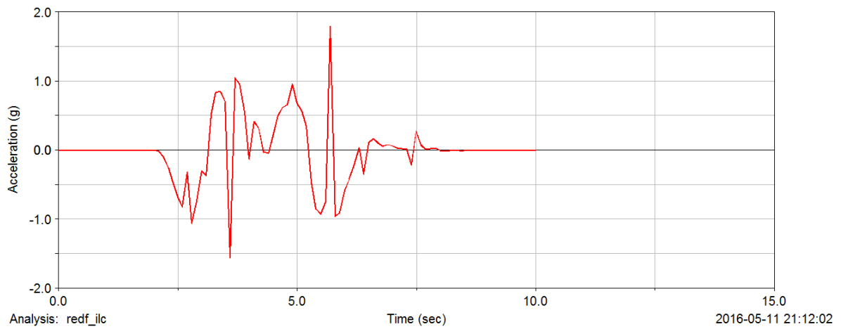
Př. 11 Boční zrychlení při simulaci s pohyblivým těžištěm v 80 km/h
