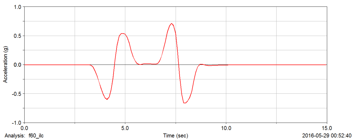
Př. 5 Boční zrychlení při simulaci v 60 km/h
