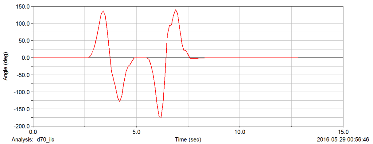
Př. 8 Úhel natočení volantu při simulaci v 70 km/h
