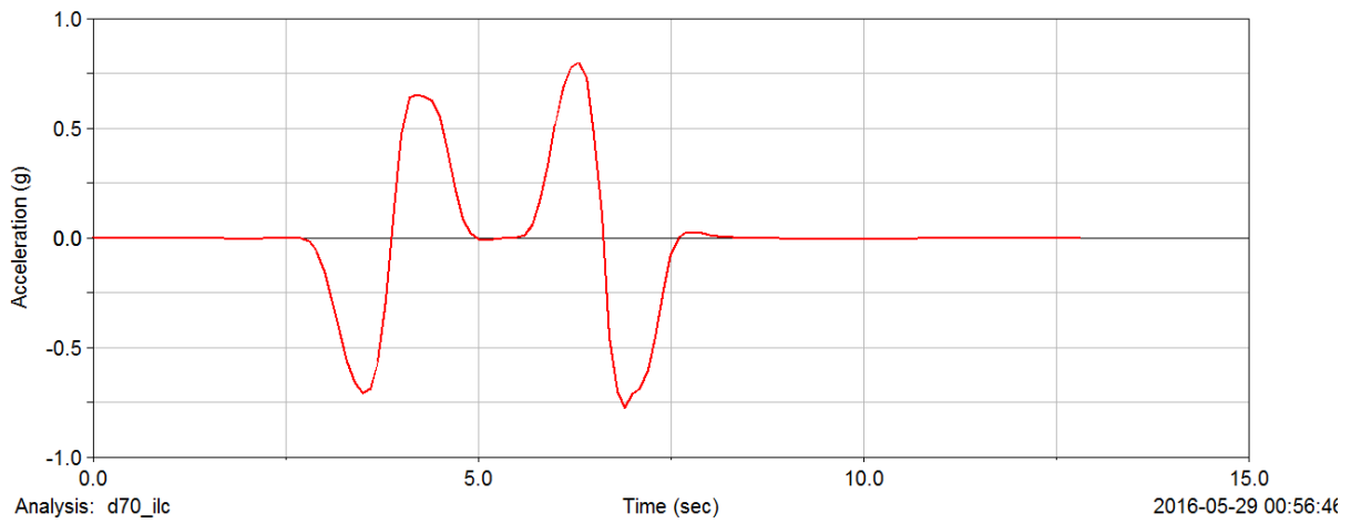
Př. 7 Boční zrychlení při simulaci v 70 km/h
