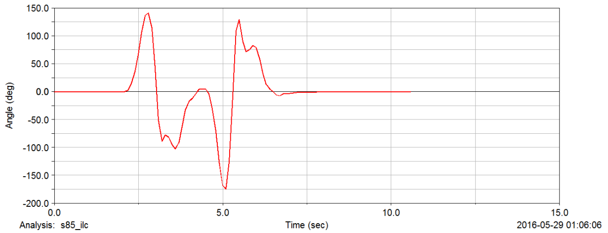
Př. 10 Úhel natočení volantu při simulaci v 85 km/h
