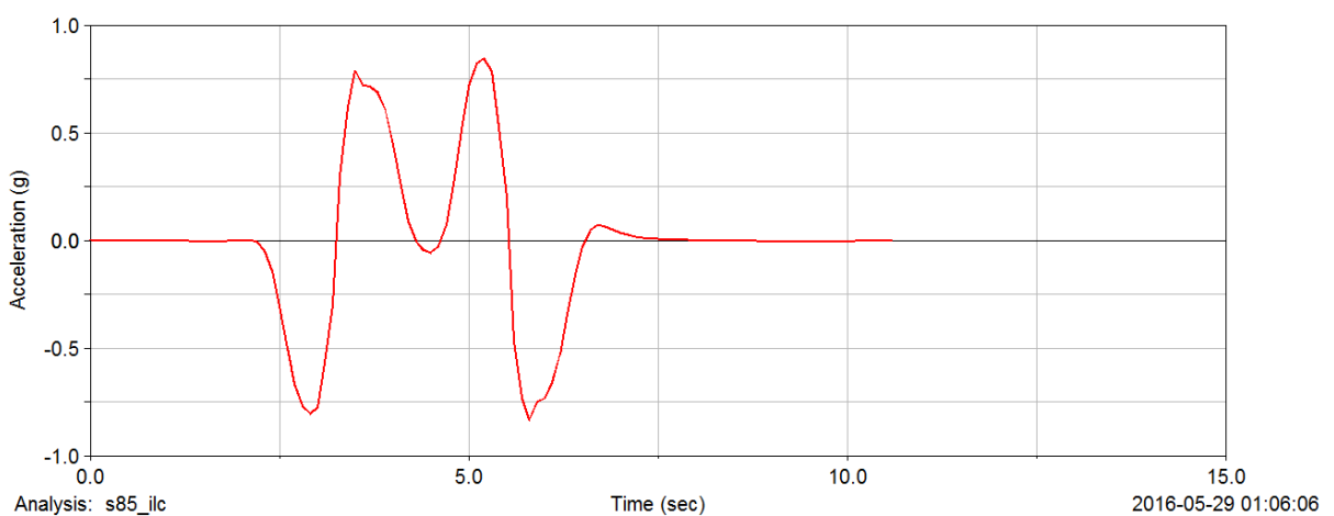
Př. 9 Boční zrychlení při simulaci v 85 km/h
