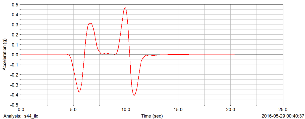
Př. 1 Boční zrychlení při simulaci v 44 km/h
