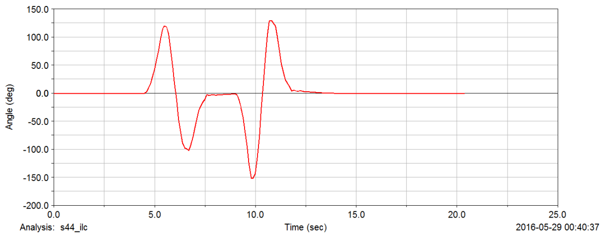
Př. 2 Úhel natočení volantu při simulaci v 44 km/h
