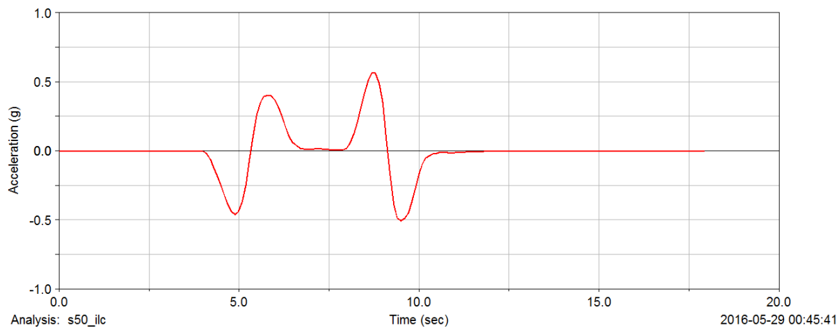
Př. 3 Boční zrychlení při simulaci v 50 km/h
