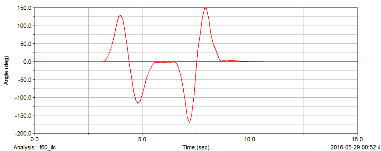
Př. 6 Úhel natočení volantu při simulaci v 60 km/h
