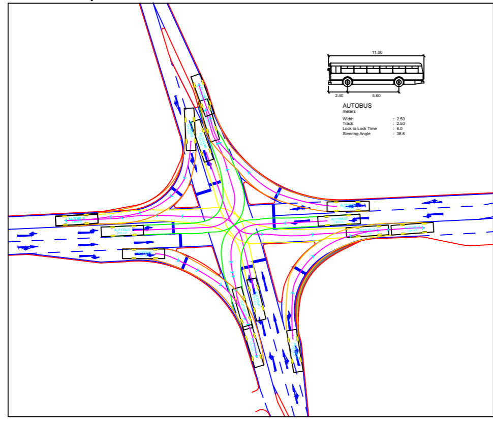
Situace obalových křivek 1:1000
