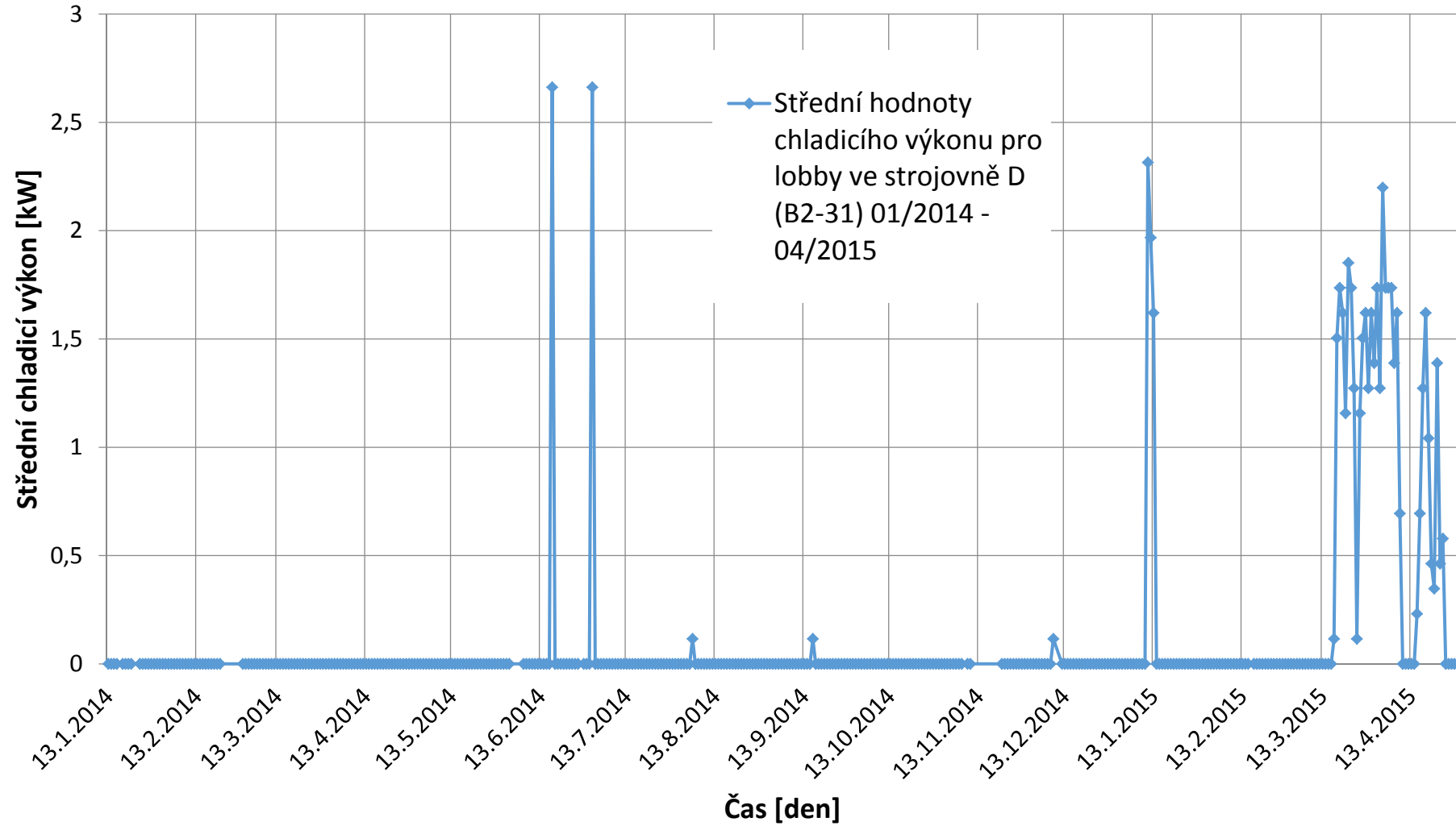
Obr. 8.5 – Střední hodnoty chladicího výkonu pro lobby ve strojovně D (B2-31)
