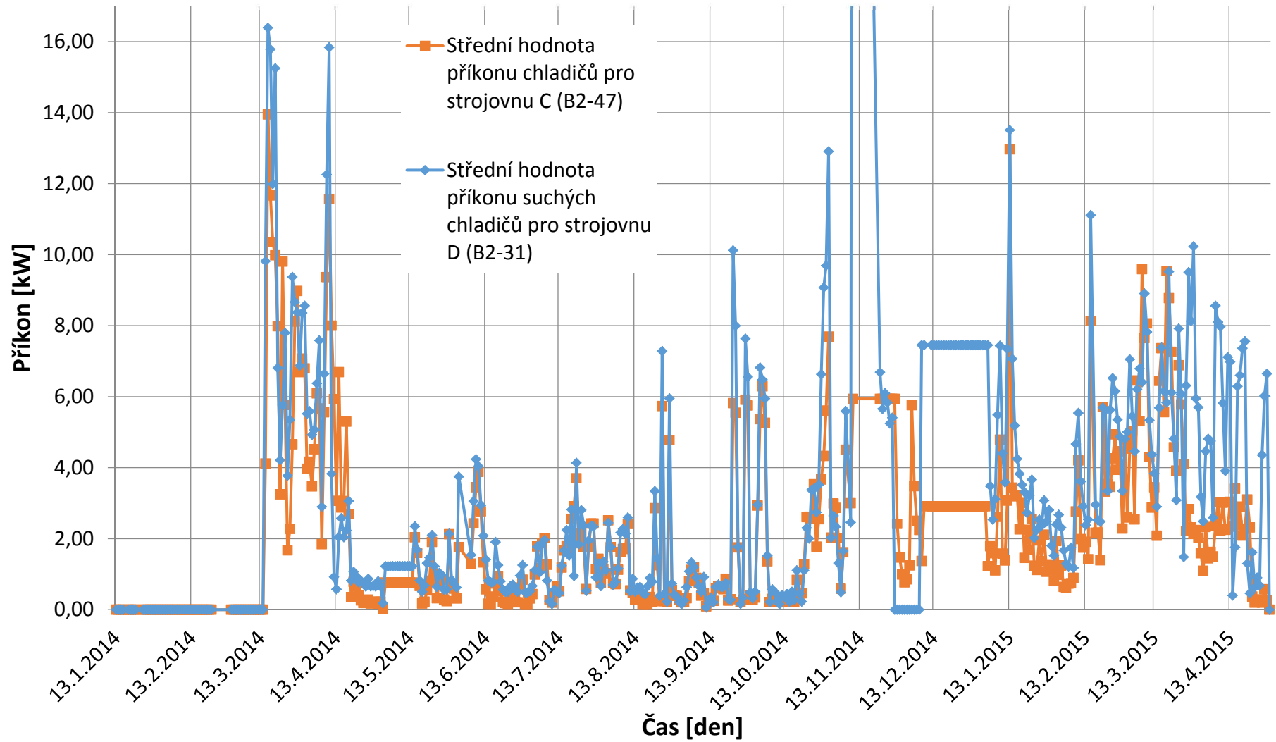
Obr. 8.23 – Střední hodnoty příkonu suchých chladičů pro jednotky ve strojovnách C a D
