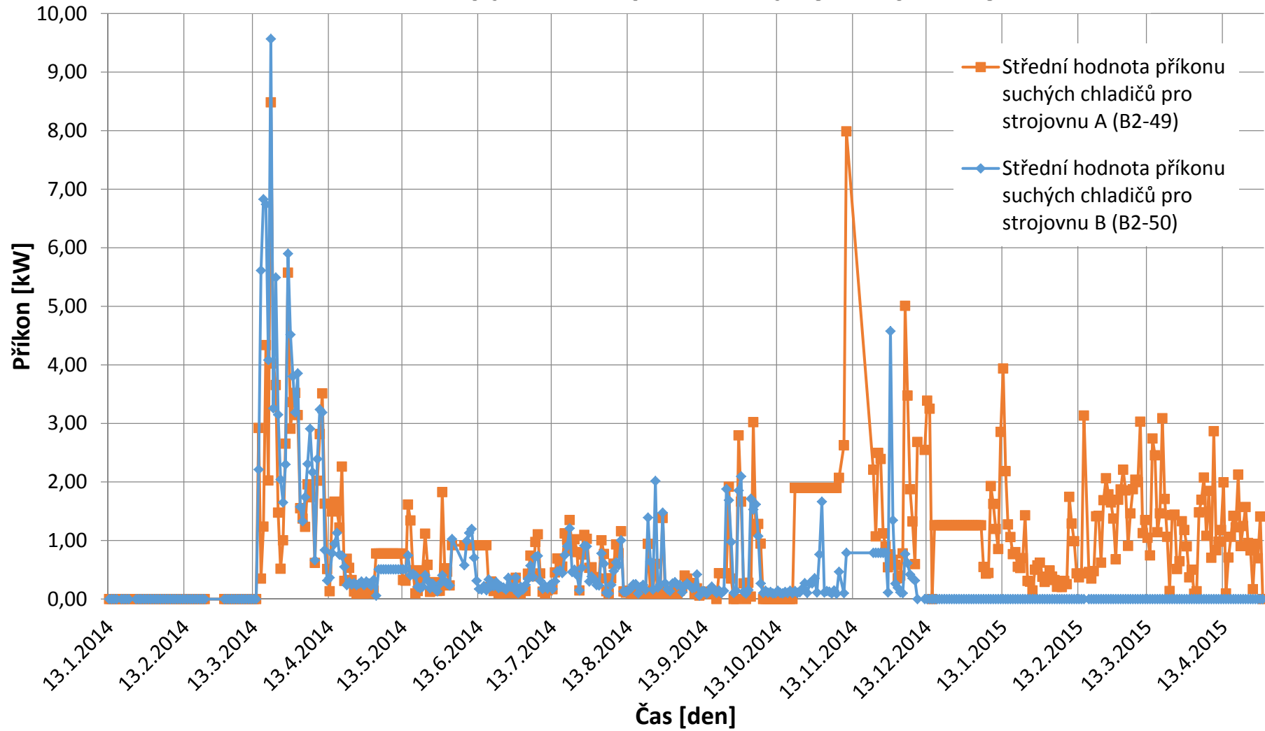
Obr. 8.22 – Střední hodnoty příkonu suchých chladičů pro jednotky ve strojovnách A a B
