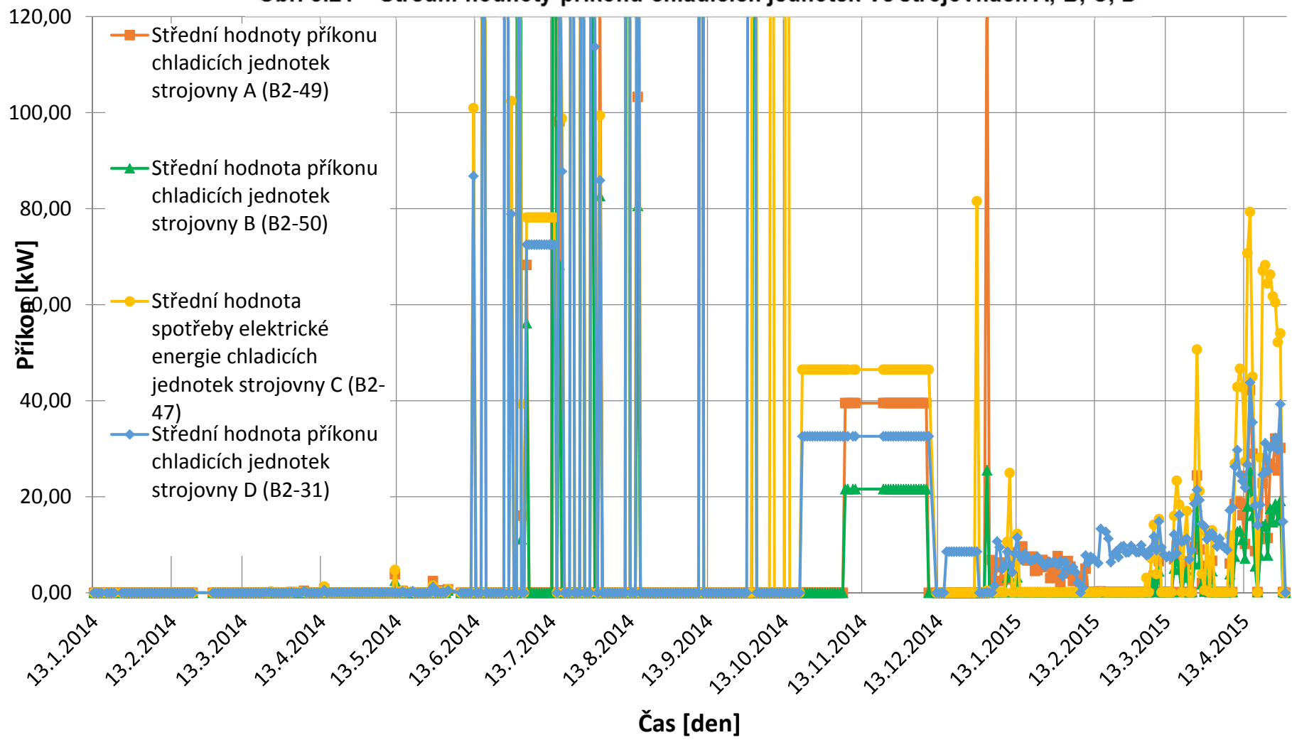
Obr. 8.21 – Střední hodnoty příkonu chladicích jednotek ve strojovnách A, B, C, D
