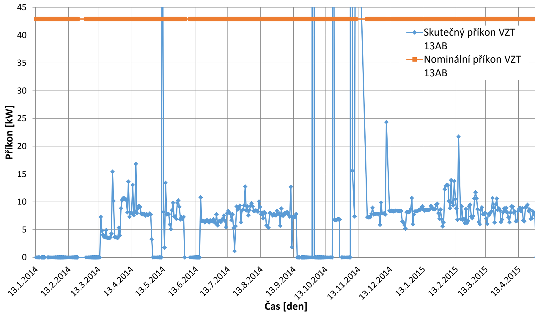
Obr. 8.18 – Skutečný a nominální příkon vzduchotechnické jednotky 13AB
