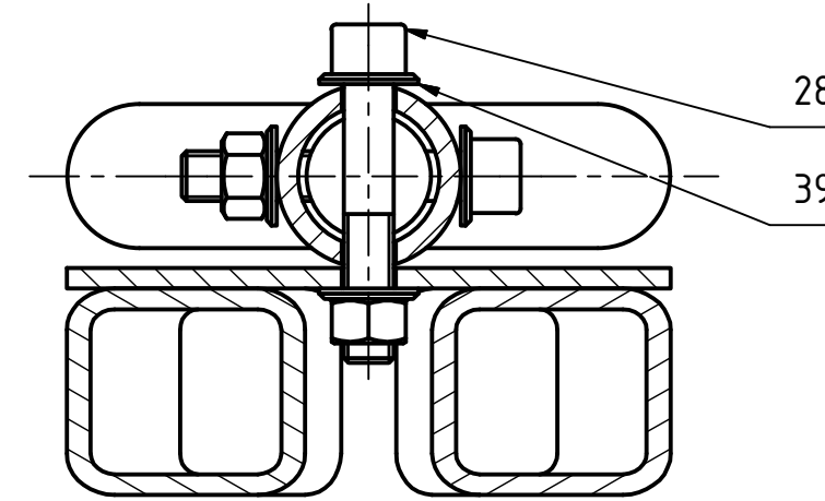
B-B (1:2)
