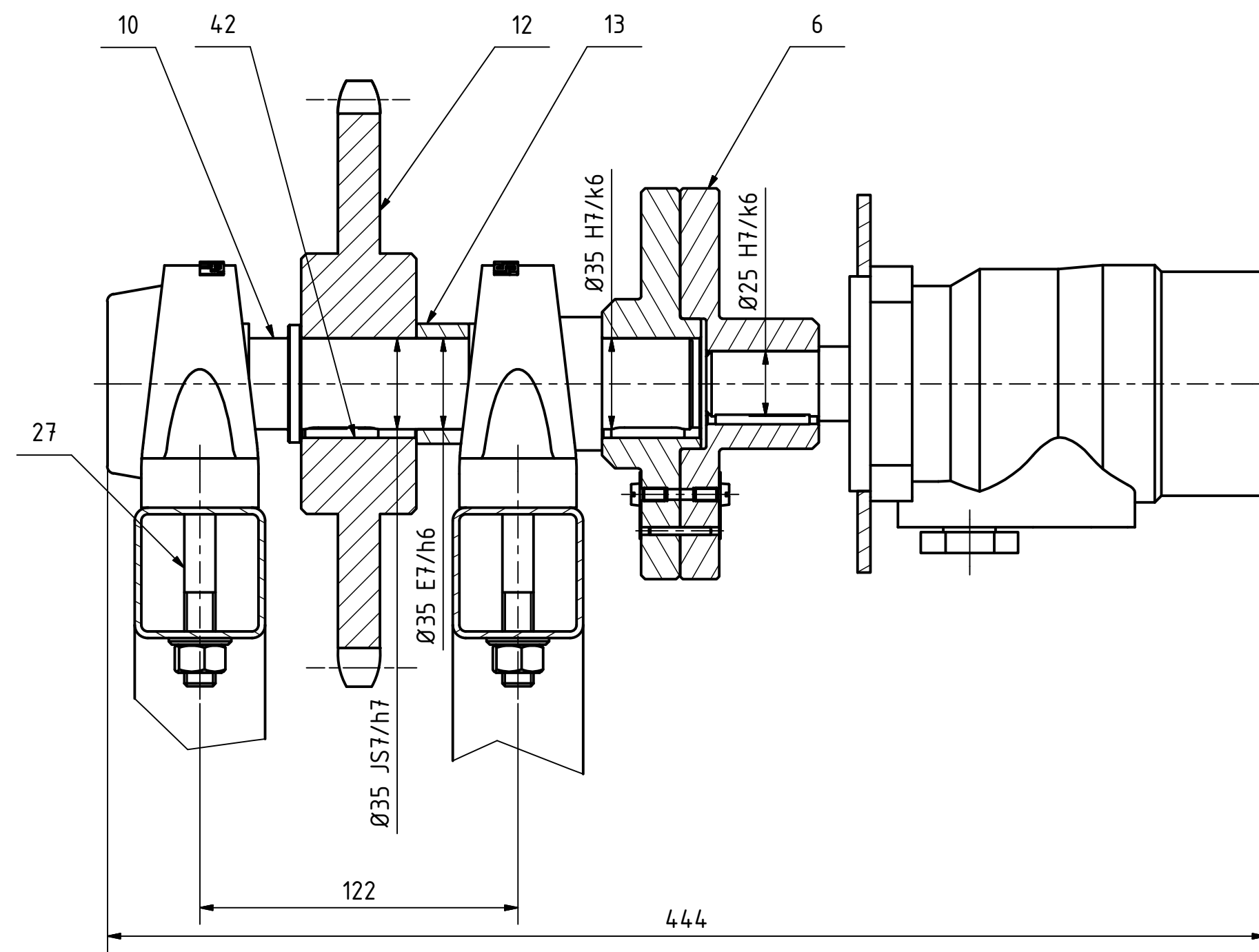
D-D (1:2)
