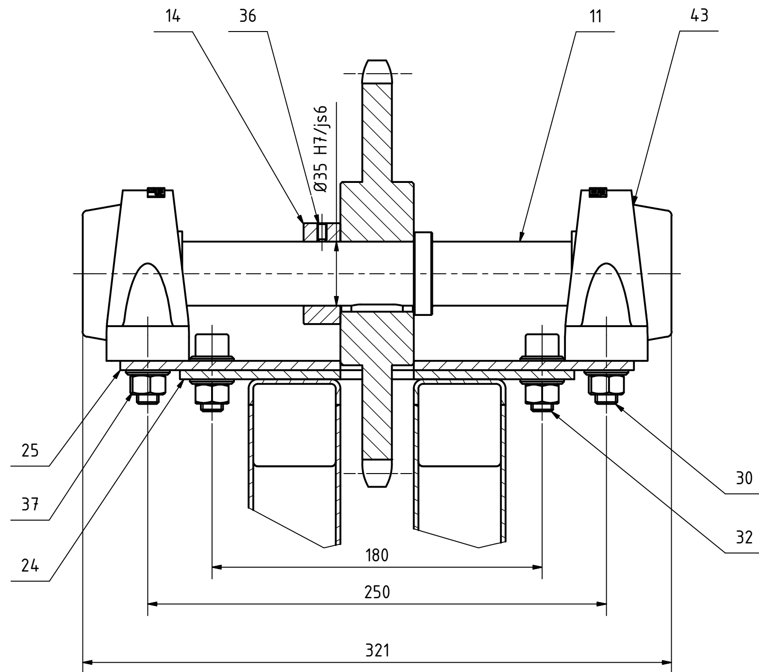
C-C (1:2)
