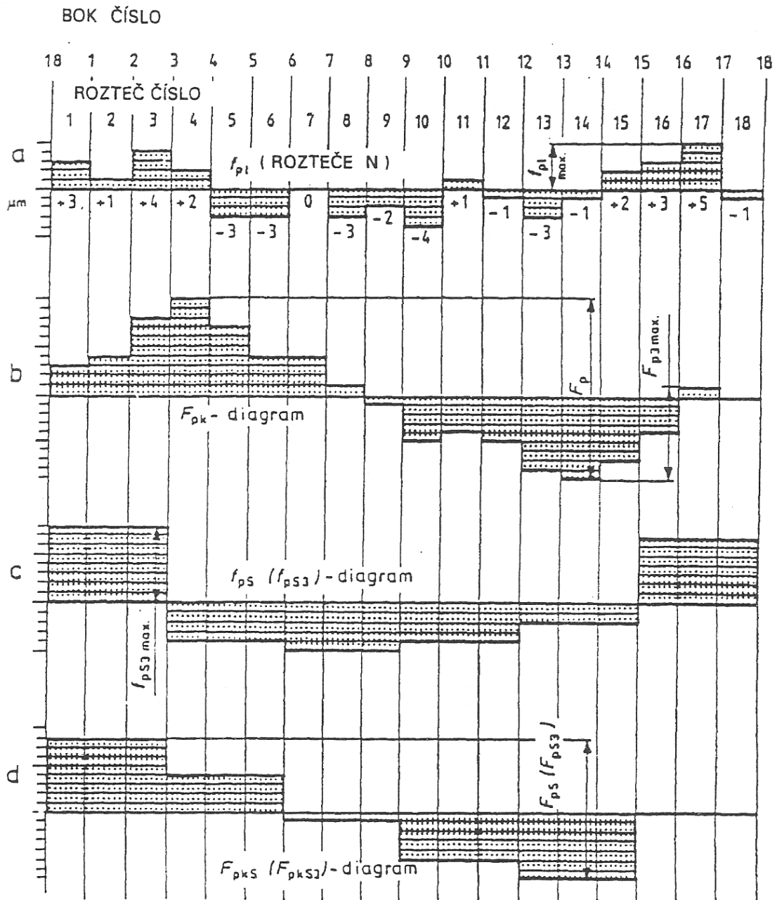
Příloha 3: Diagram průběhu úchylek čelních roztečí [27].
