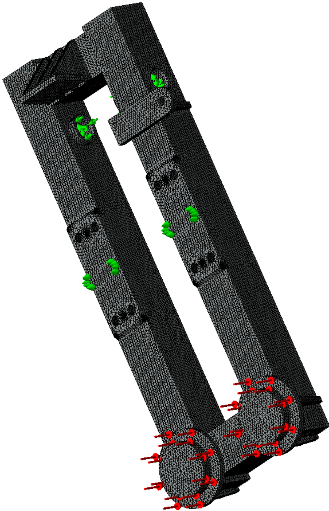
Příloha 2. Model kyvné vidlice s vytvořenou sítí pro pevnostní kontrolu metodou konečných prvků
