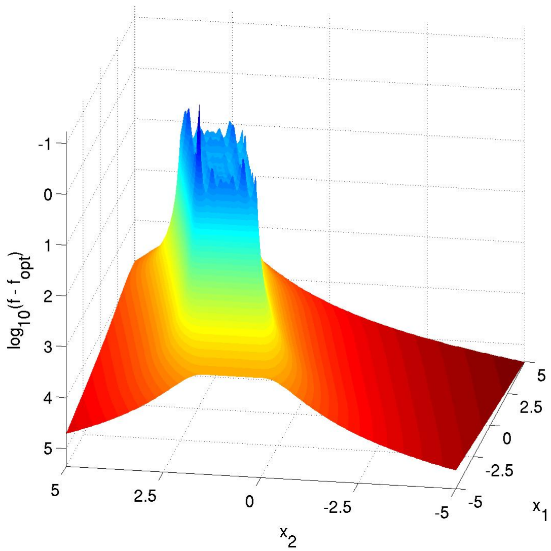
Obrázek A.20: Funkce 20 (Schwefel Function)
