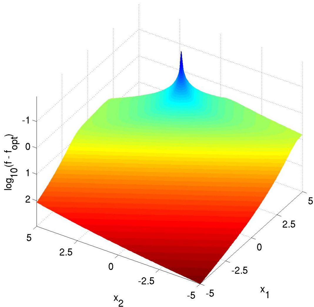
Obrázek A.14: Funkce 14 (Different Powers Function)
