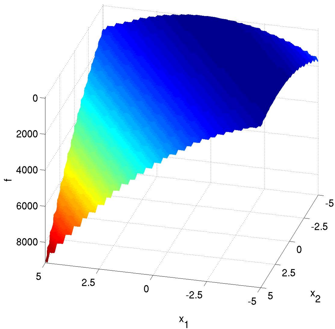
Obrázek A.7: Funkce 7 (Step Ellipsoidal Function)
