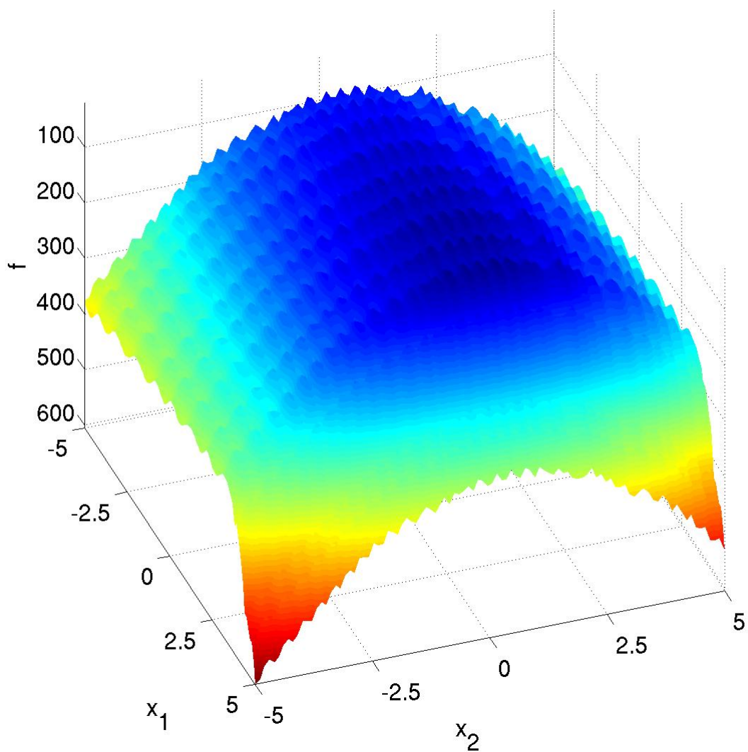
Obrázek A.4: Funkce 4 (Büche-Rastrigin Function)
