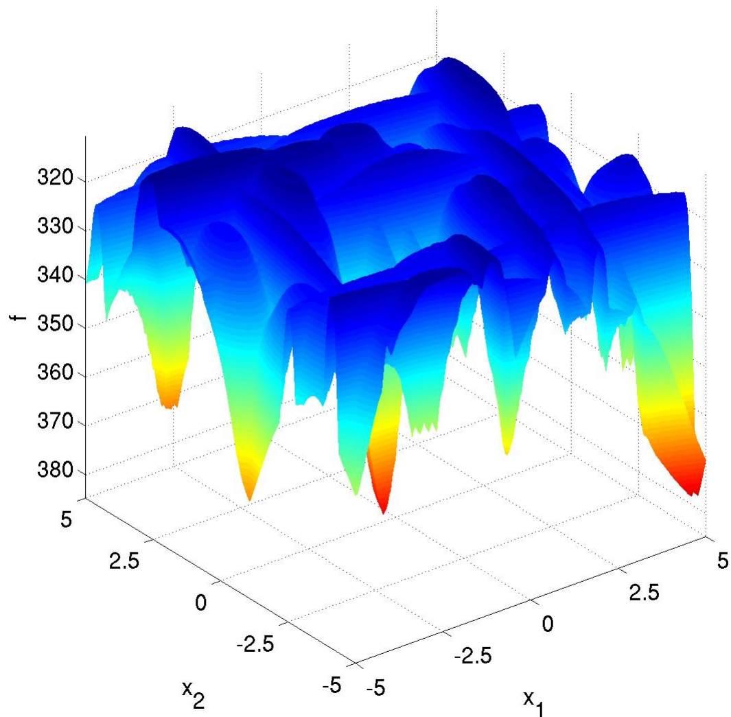
Obrázek A.21: Funkce 21 (Gallagher's Gaussian 101-me Peaks Function)
