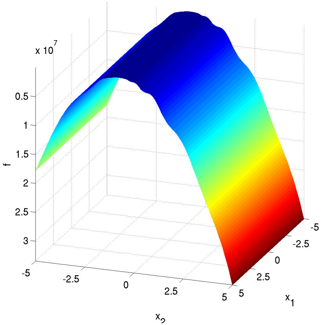
Obrázek A.2: Funkce 2 (Ellipsoidal Function)
