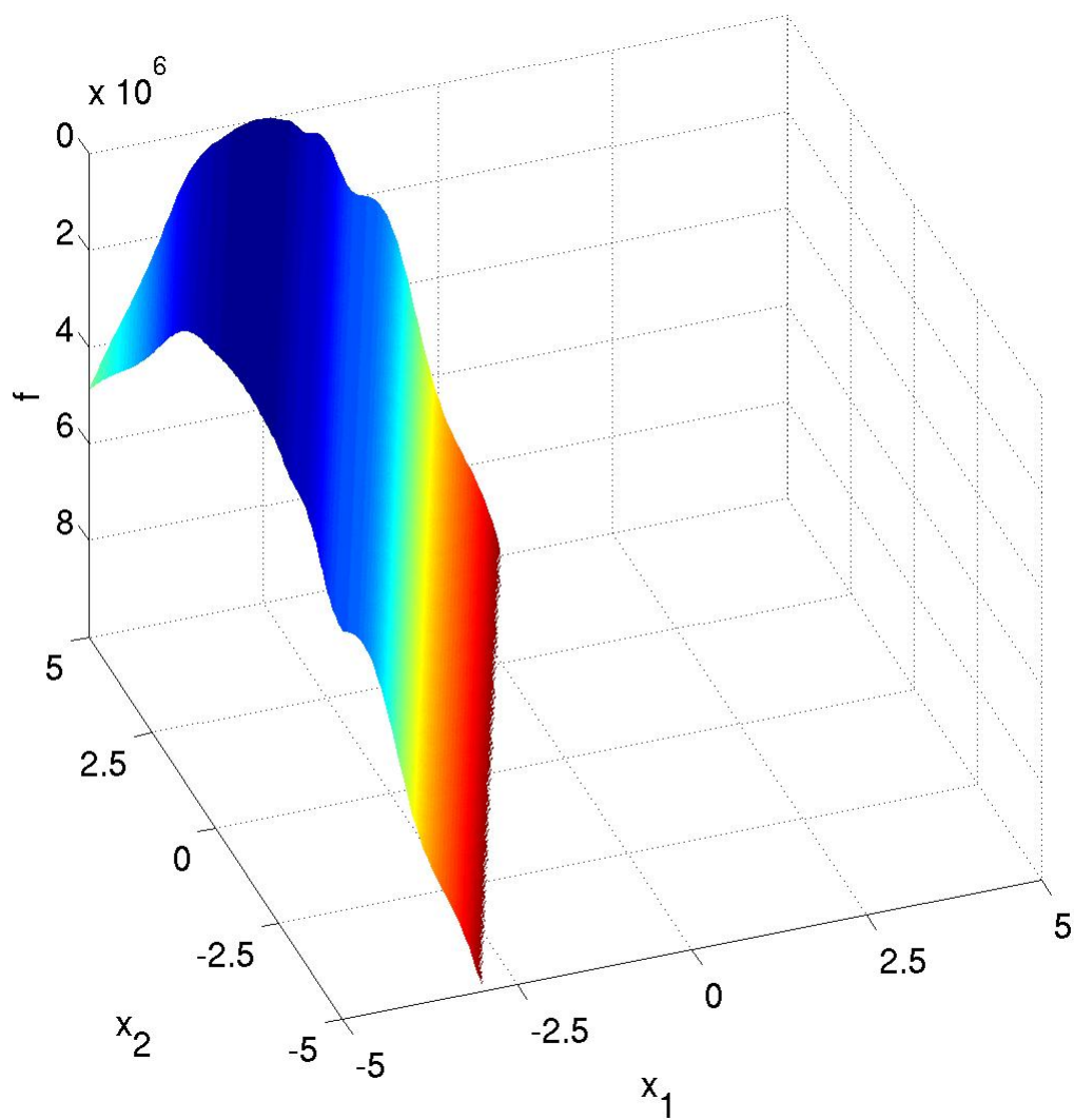
Obrázek A.11: Funkce 11 (Discus Function)
