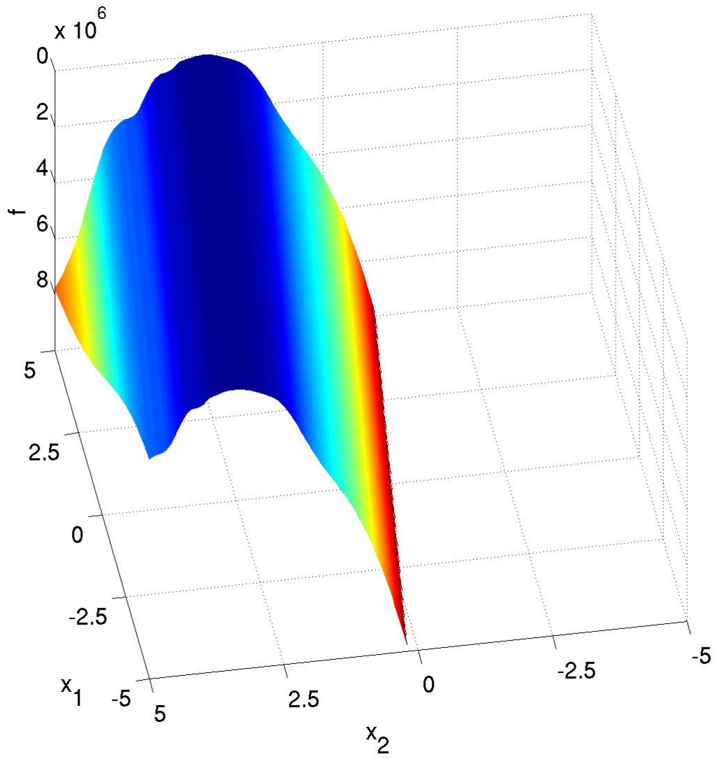
Obrázek A.10: Funkce 10 (Ellipsoidal function)
