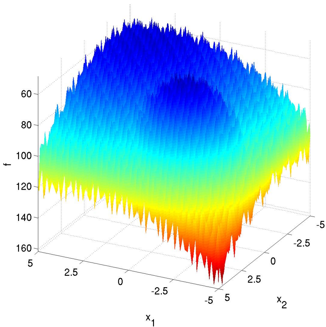
Obrázek A.24: Funkce 24 (Lunacek bi-Rastrigin Function)
