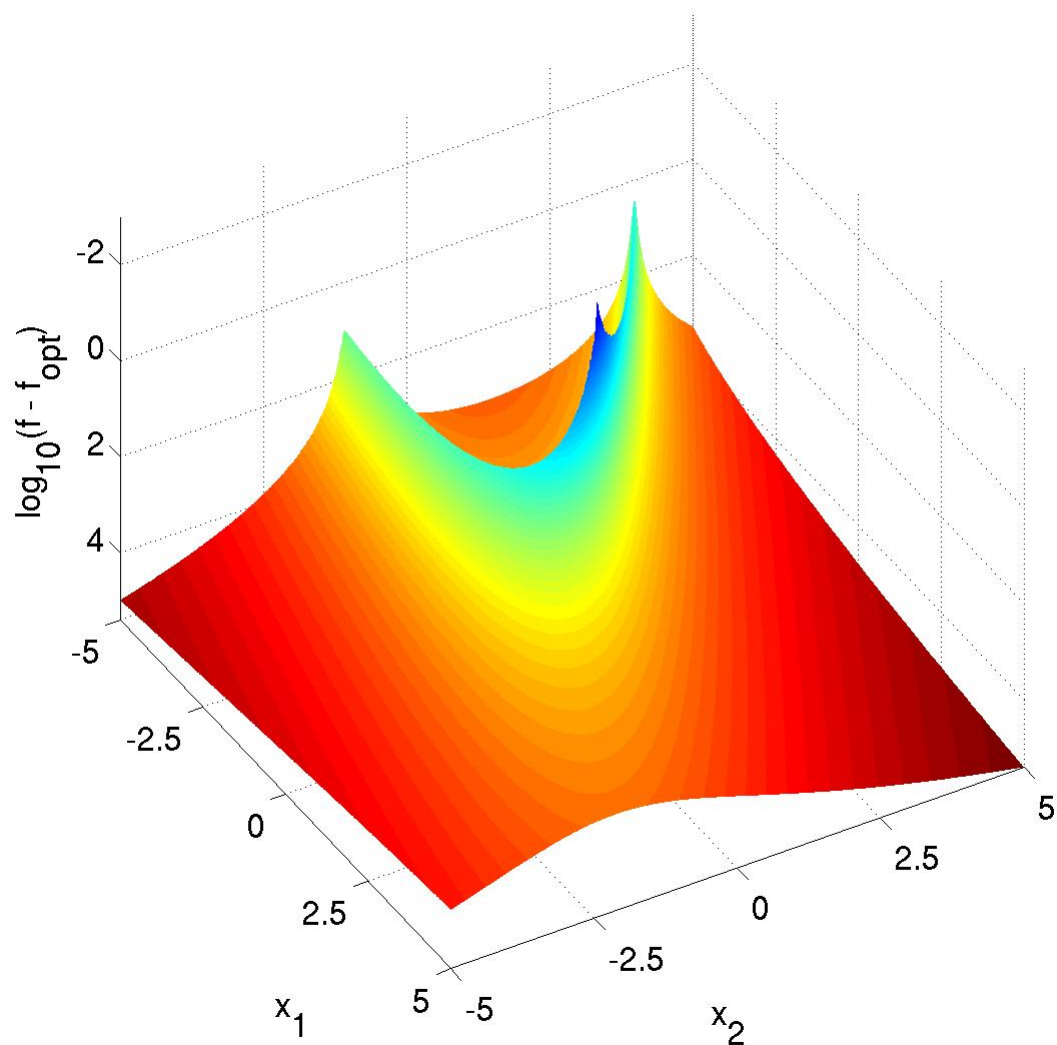
Obrázek A.9: Funkce 9 (Rosenbrock Function, rotated)
