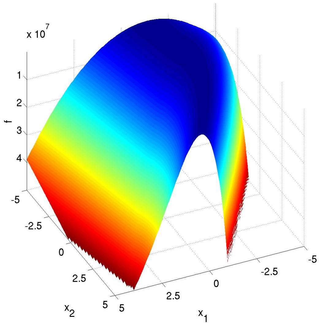
Obrázek A.12: Funkce 12 (Bent Cigar Function)
