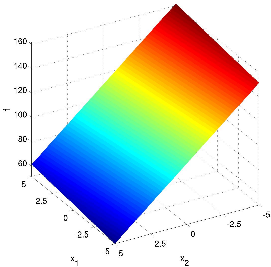
Obrázek A.5: Funkce 5 (Linear Slope)
