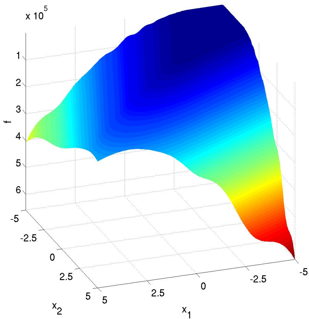
Obrázek A.6: Funkce 6 (Attractive Sector Function)
