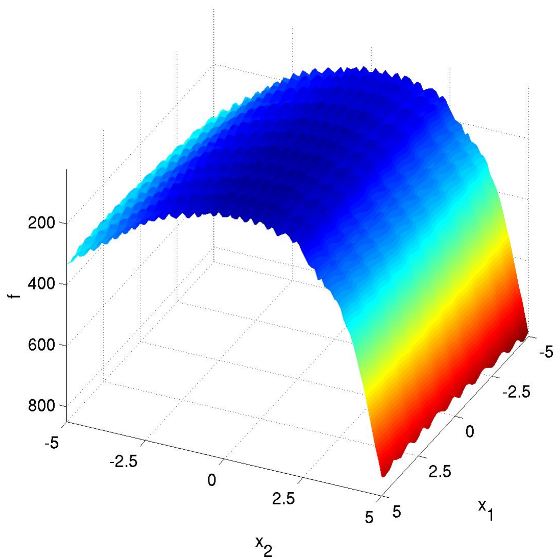
Obrázek A.3: Funkce 3 (Rastrigin Function)
