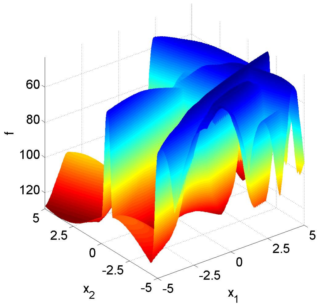
Obrázek A.22: Funkce 22 (Gallagher's Gaussian 21-hi Peaks Function)
