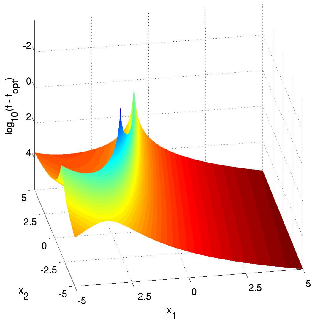
Obrázek A.8: Funkce 8 (Step Ellipsoidal Function)
