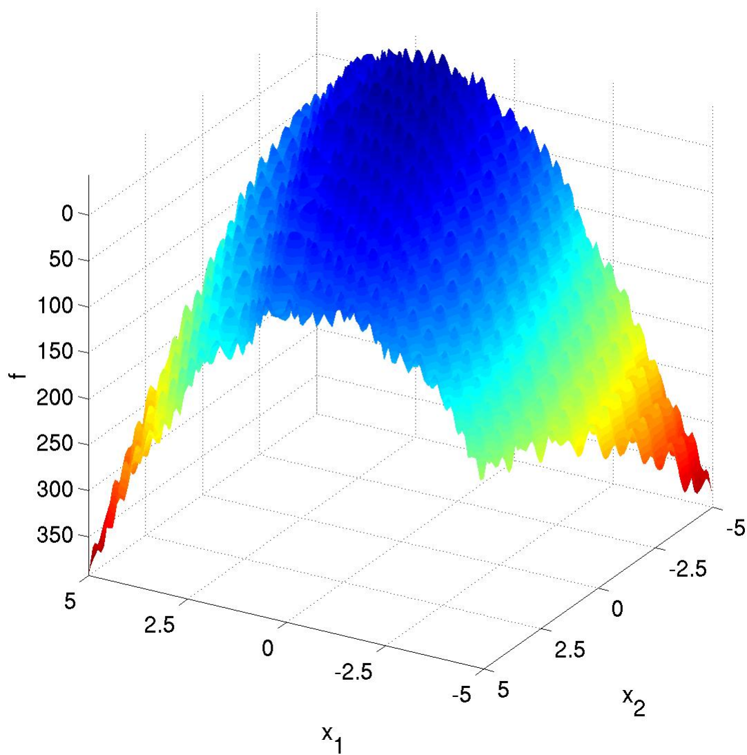
Obrázek A.15: Funkce 15 (Rastrigin Function)
