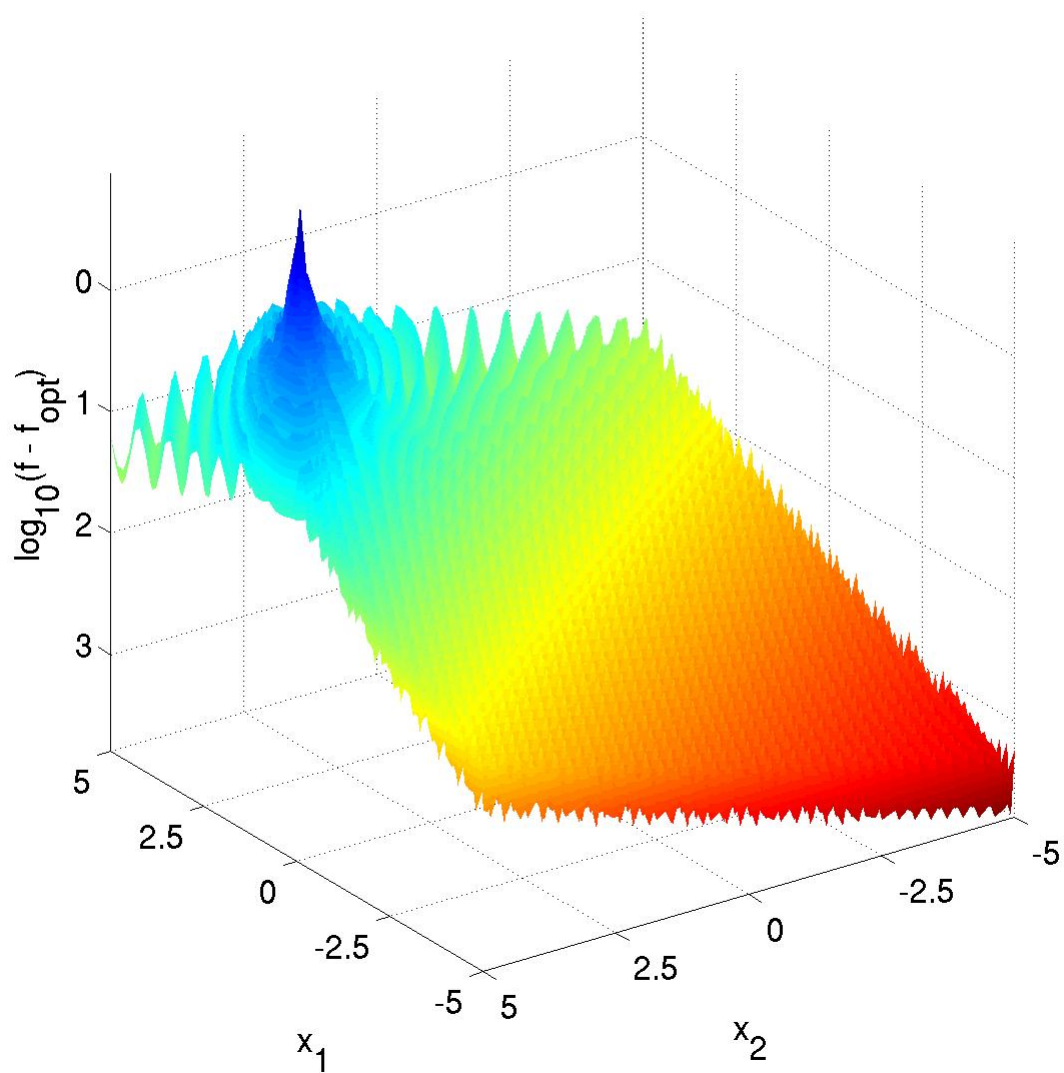
Obrázek A.17: Funkce 17 (Schaffers F7 Function)
