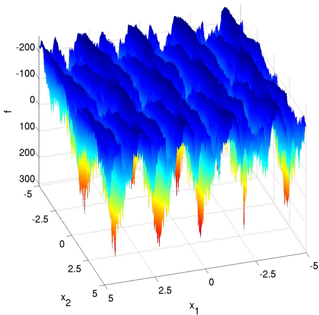
Obrázek A.16: Funkce 16 (Weierstrass Function)
