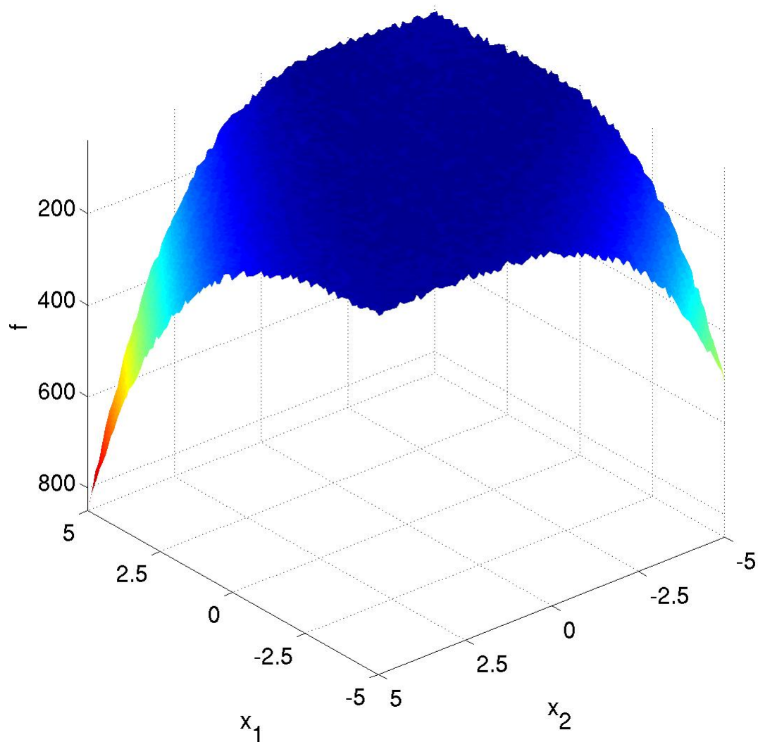
Obrázek A.19: Funkce 19 (Composite Griewank-Rosenbrock Function F8F2)
