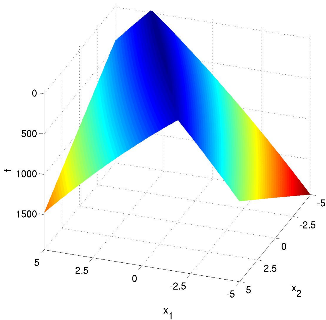
Obrázek A.13: Funkce 13 (Sharp Ridge Function)
