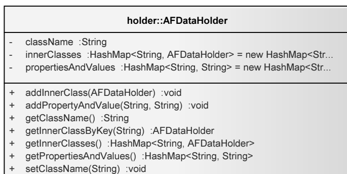
Obrázek 4.4: Třída, která reprezentuje data ve formuláři, na jejím základě je sestaven objekt, který je odeslán na server.
