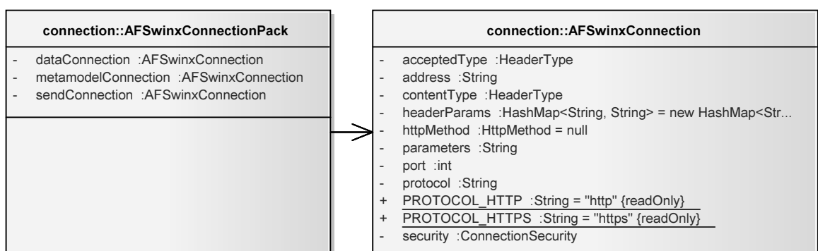
Obrázek 4.2: Třídy zodpovědné za specifikaci zdrojů a způsobu připojení.
