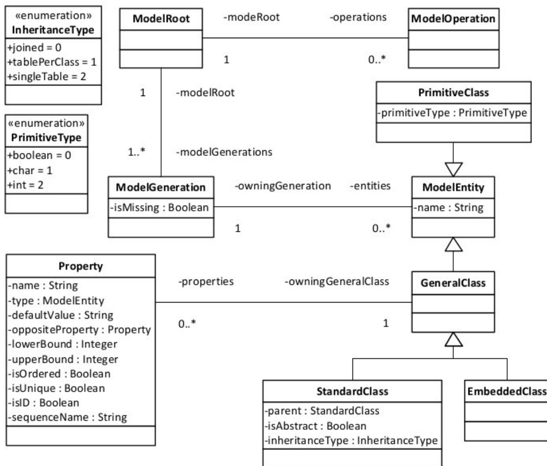
Obrázek 3.2: Aplikační metamodel v průběhu vývoje obrázků převzat z [Jez12]
