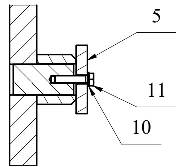
B-B (1 : 5)
