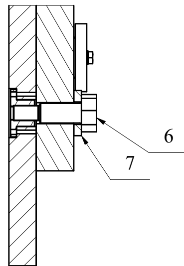
B-B (1 : 5)
