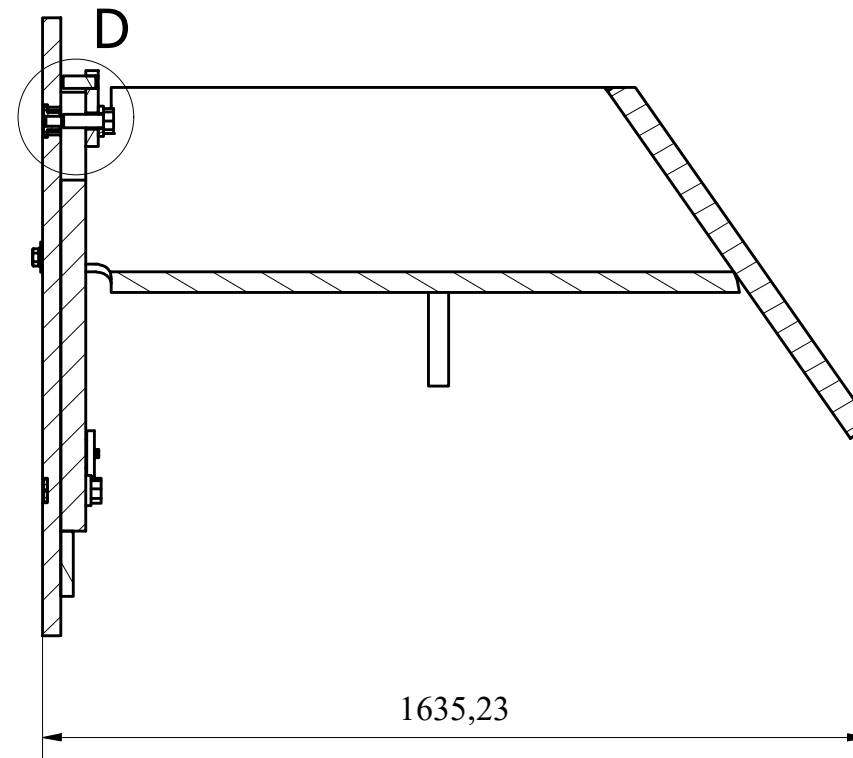
C-C (1 : 15)
