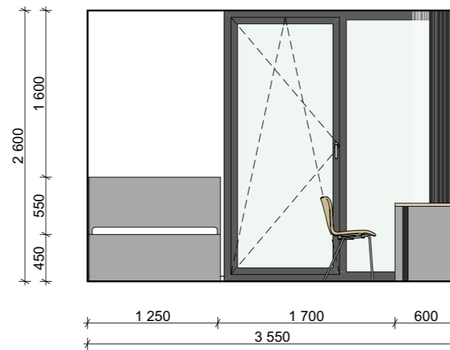
POHLED 03
