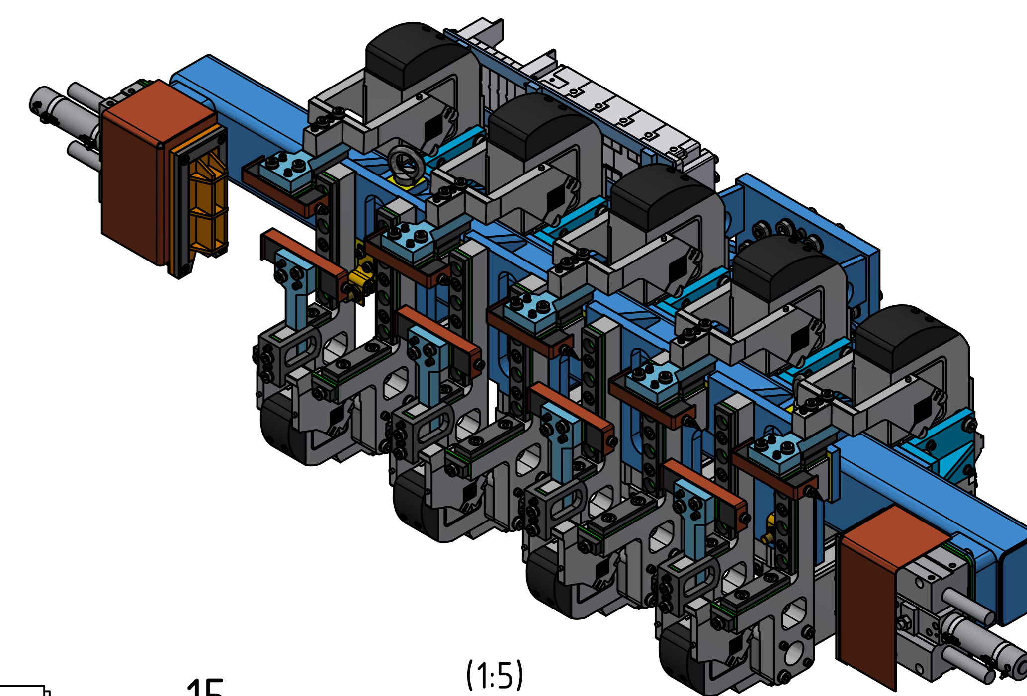
POZICE TĚŽIŠTĚ 365 mm OD PŘÍPOJNÉHO ROZHRANÍ (PŘÍRUBA)
