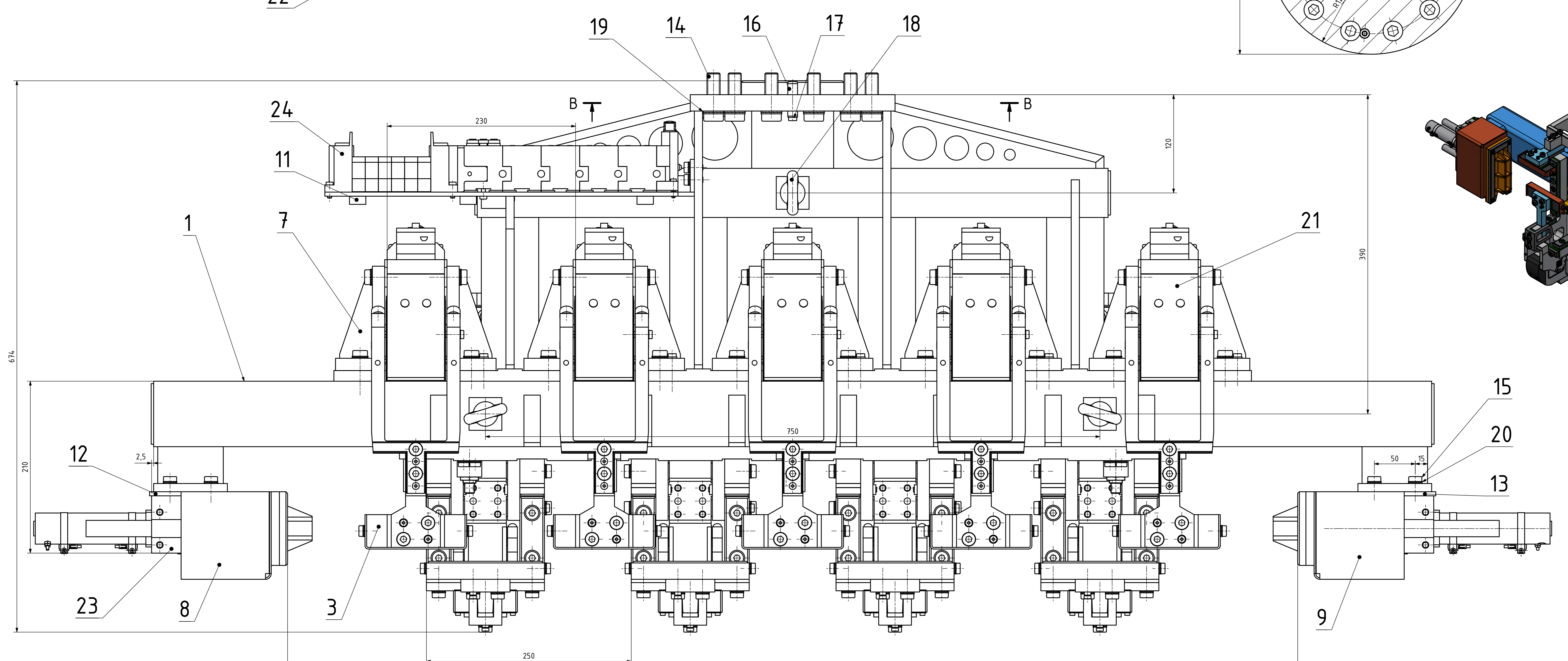
POZICE TĚŽIŠTĚ 365 mm OD PŘÍPOJNÉHO ROZHRANÍ (PŘÍRUBA)
