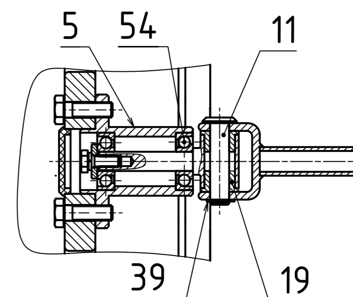
B-B (1:2)
