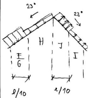
PŘÍČNÝ SCHEMA
