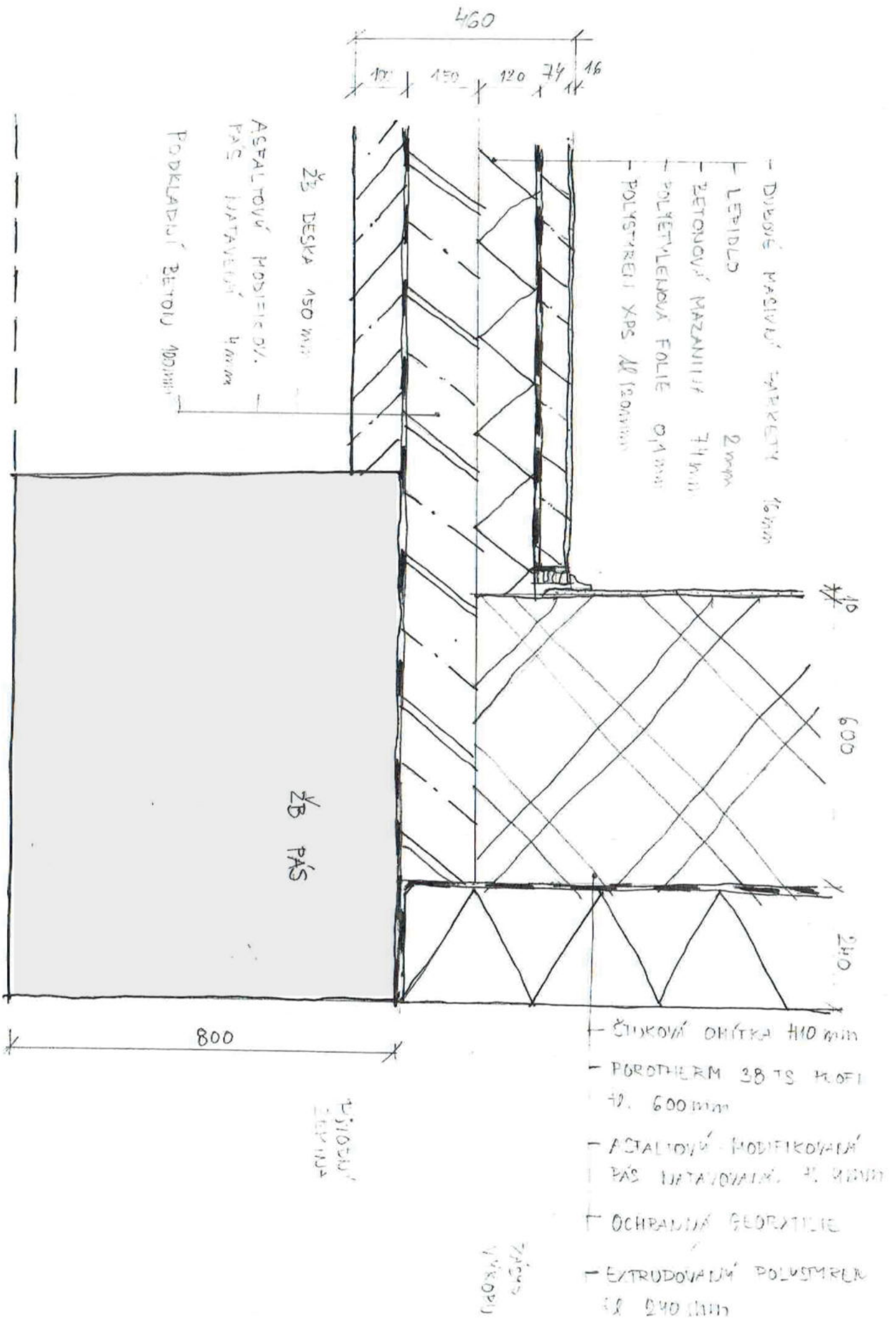
D2 DETAIL ZÁKLADU NOVÝ M: 1:10
