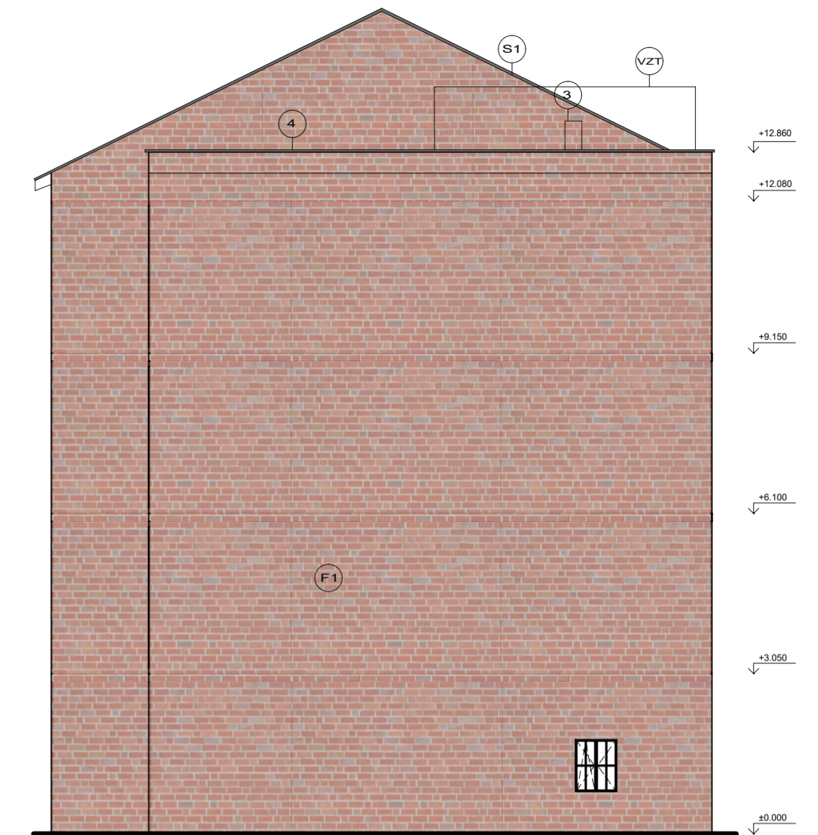
POHLED JIH
