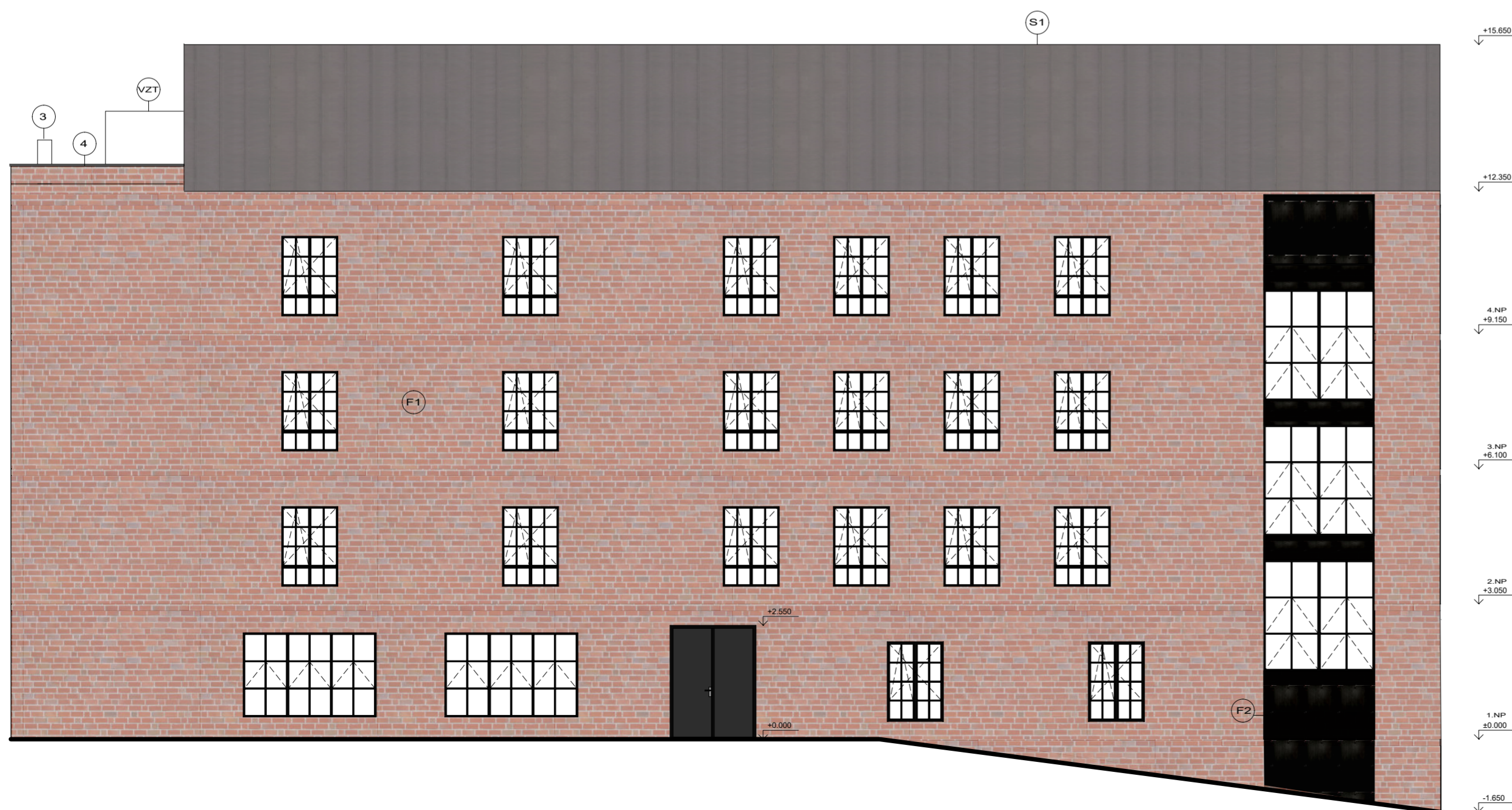
POHLED VÝCHOD
