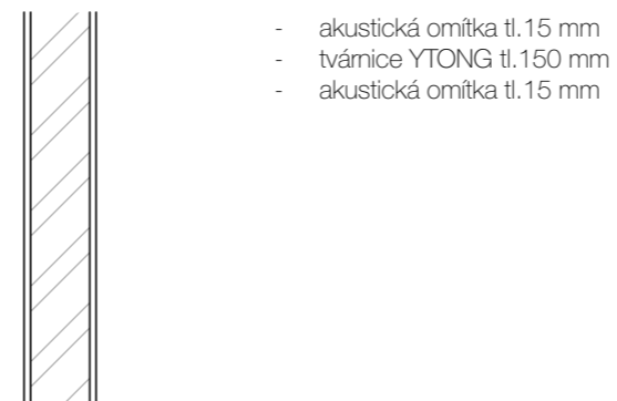
Z3 - zděná příčka tl.150mm bytová
