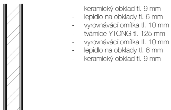
Z5 - zděná příčka tl.150mm koupelna/WC
