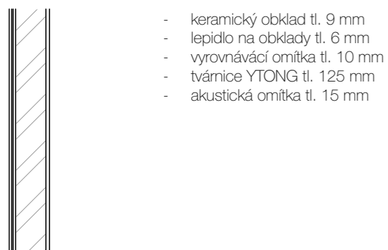
Z9 - zděná příčka tl.150mm koupelna/byt
