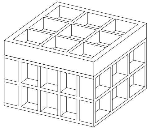
P - 4 STOJAN NA VINYLOVÉ DESKY 1 300 x 1 280
