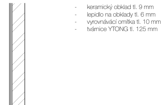
Z4 - zděná příčka tl.125mm byt/ instalační šachta
