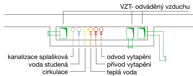
S1 TYPICKÉHO PODLAŽÍ
