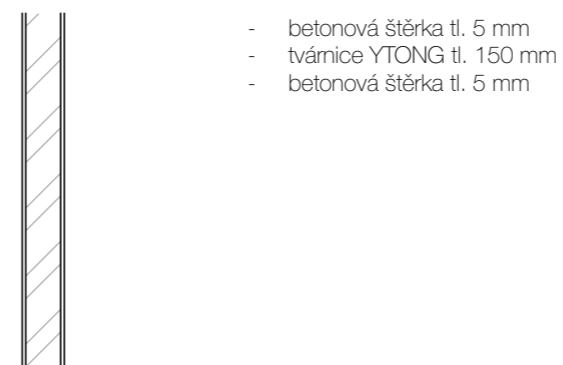
Z7 - zděná příčka tl.150mm sklepy
