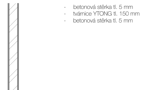
Z8 - zděná příčka tl.125mm technická místnost, kočarkárna/chodba
