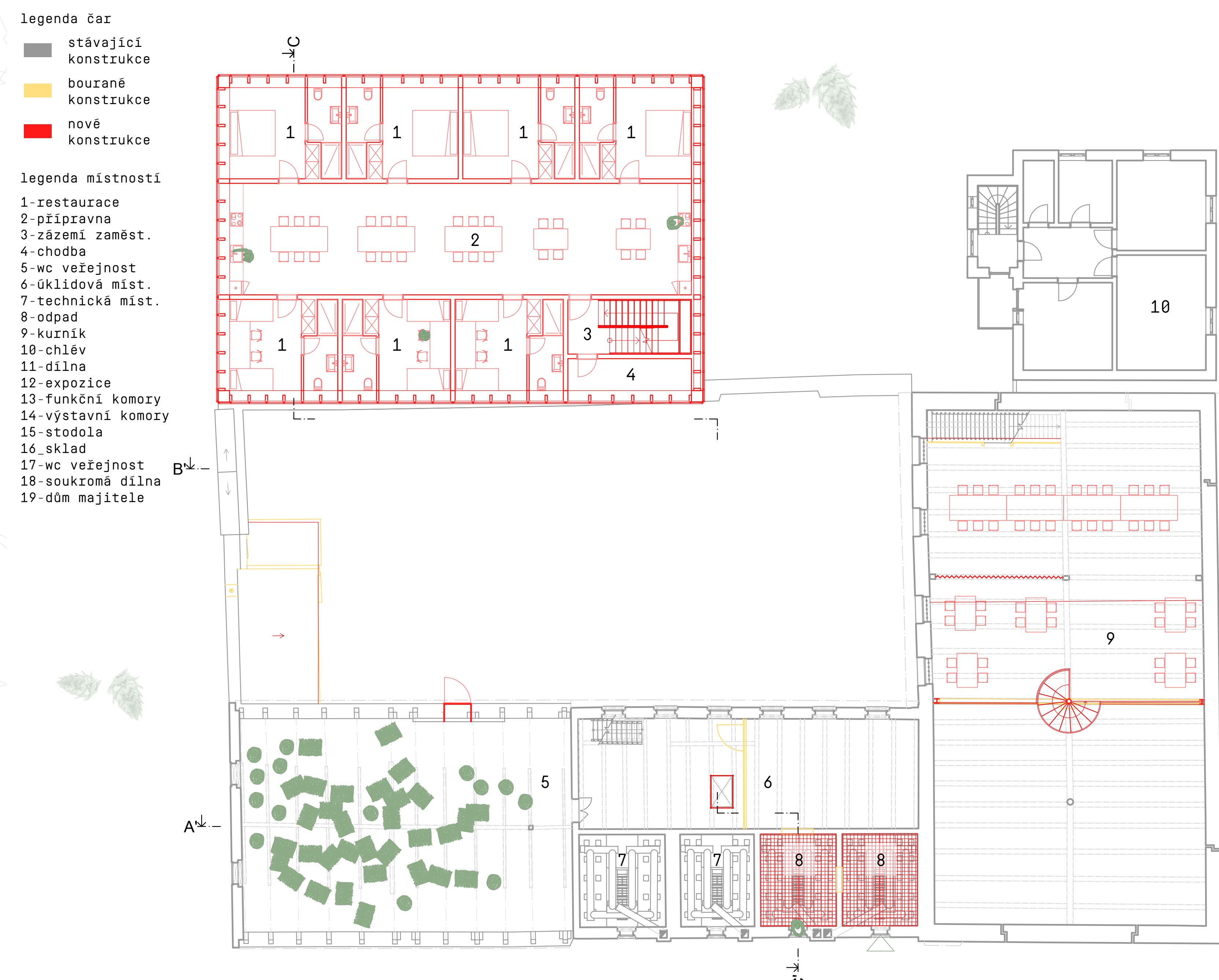
půdorys 2NP
