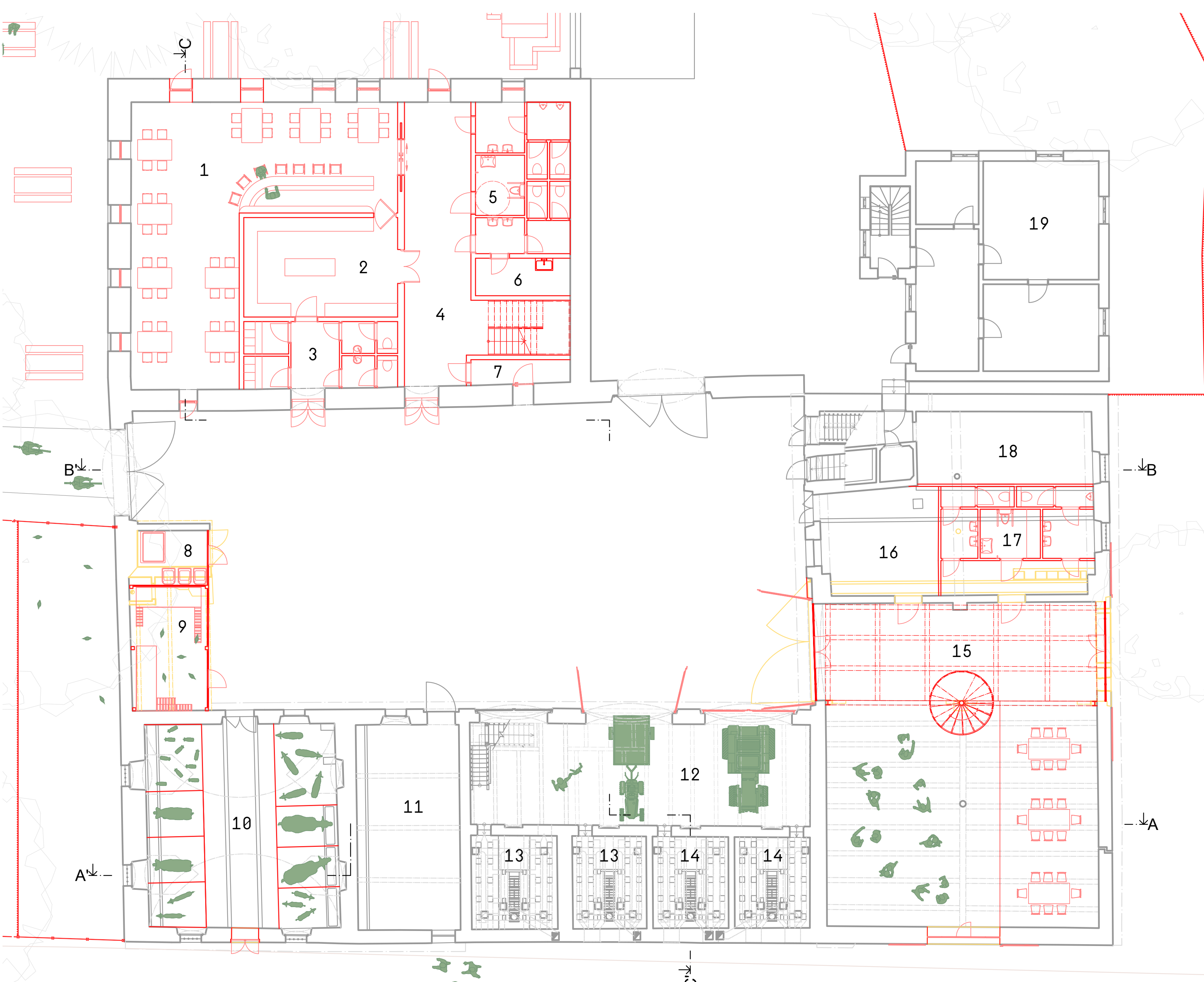
půdorys 1NP
