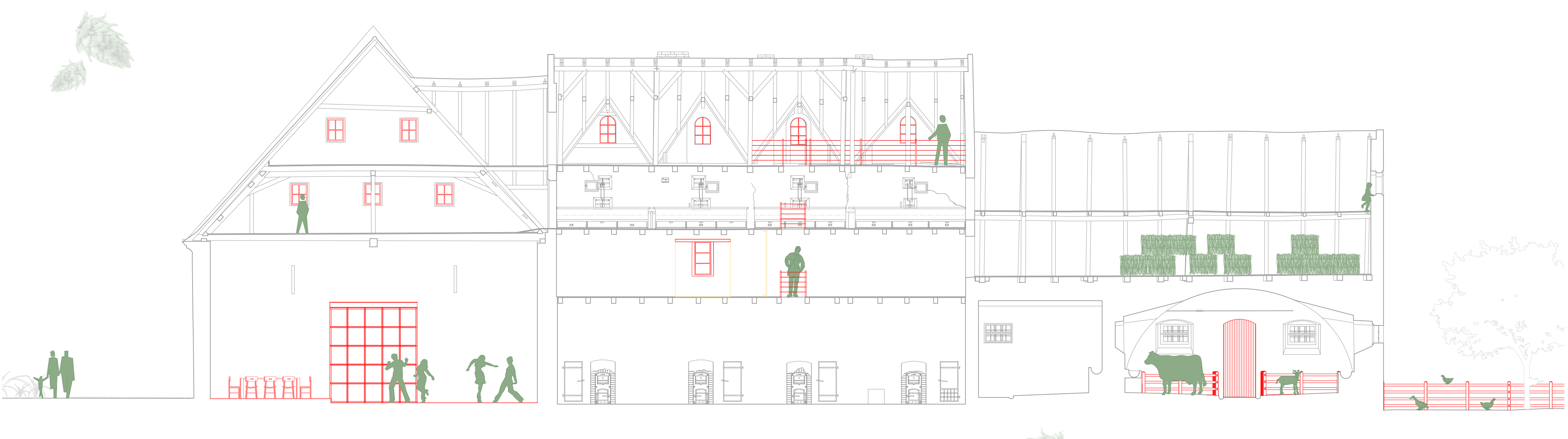
řez A-A'
