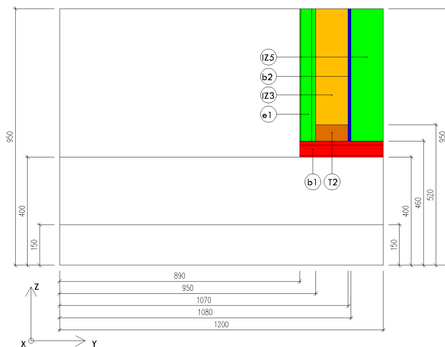
Obr. 50 Vysvětlující řez AA zkušebního tělesa ke zdrojovému kódu programu FDS
