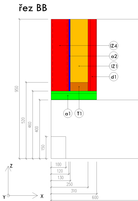
Obr. 51 Vysvětlující řez BB zkušebního tělesa ke zdrojovému kódu programu FDS
