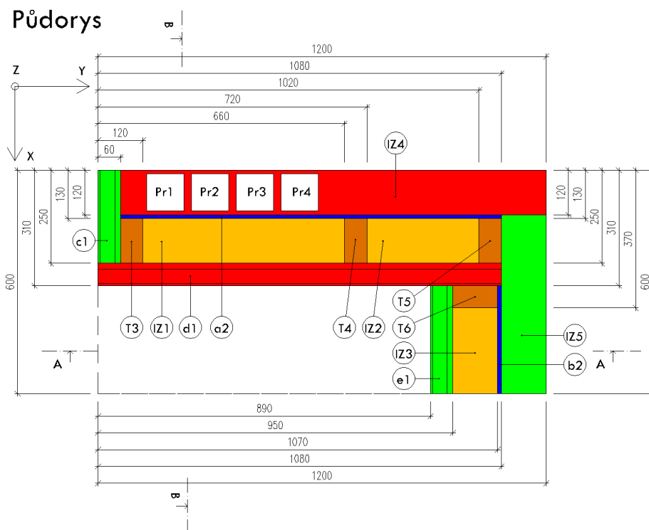
Obr. 49 Vysvětlující půdorys zkušebního tělesa ke zdrojovému kódu programu FDS
