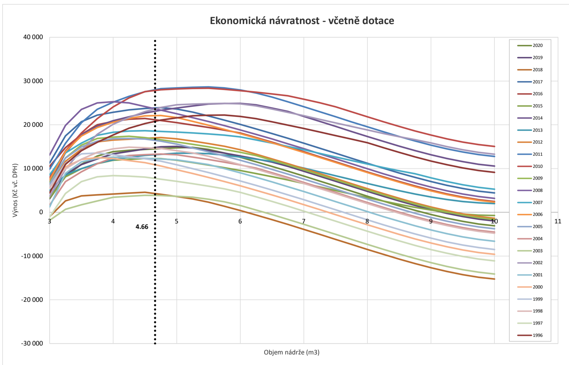
Příloha č. 9: Grafy ekonomické návratnosti různých velikostí akumulčních nádrží v letech 1996-2020 v lokalitě Žatecko v případě získání dotace a bez dotace pro KALENDÁŘNÍ metodu ovládnání závlahového systému
