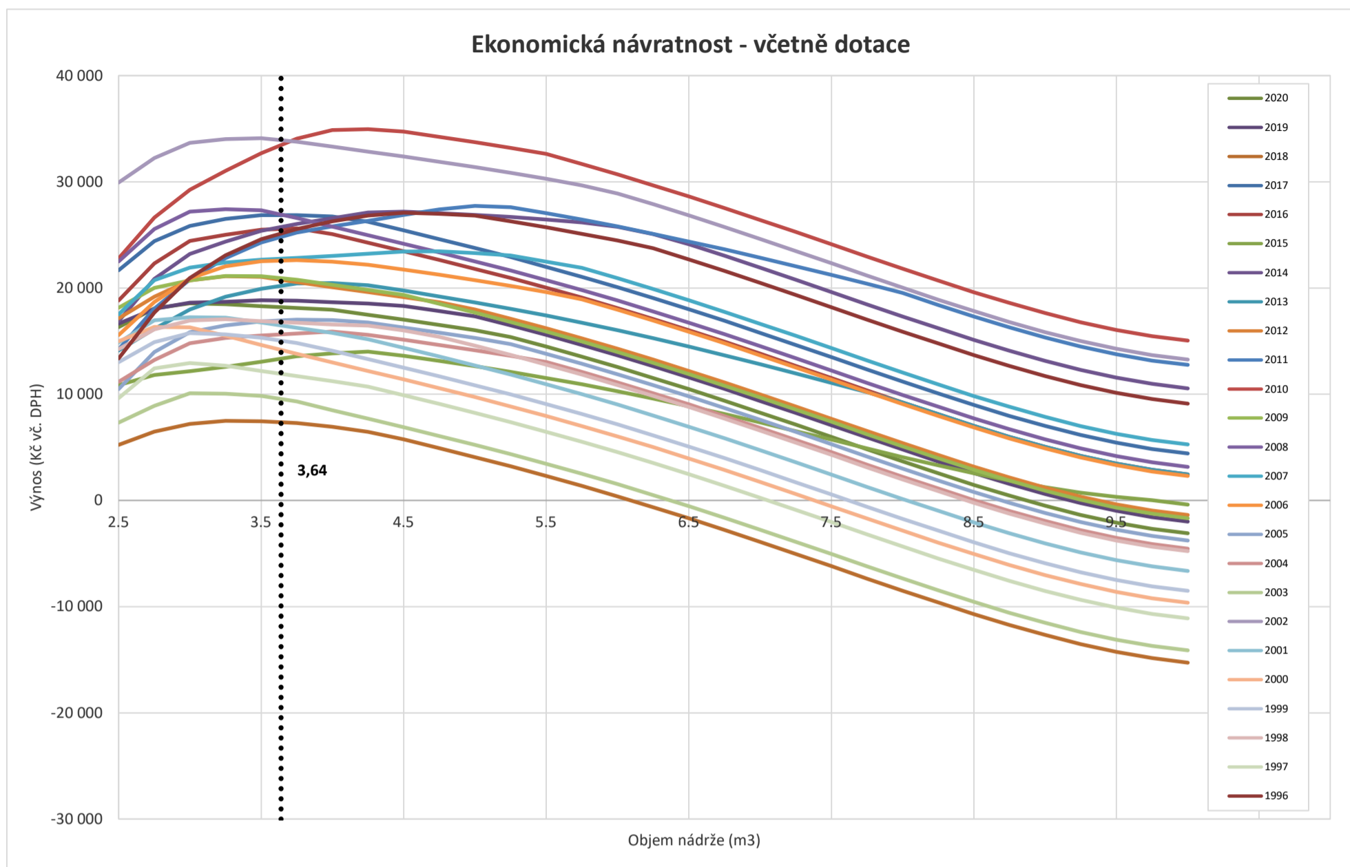
Příloha č. 10: Grafy ekonomické návratnosti různých velikostí akumulčních nádrží v letech 1996-2020 v lokalitě Žatecko v případě získání dotace a bez dotace pro INTERVALOVOU metodu ovládání závlahového systému
