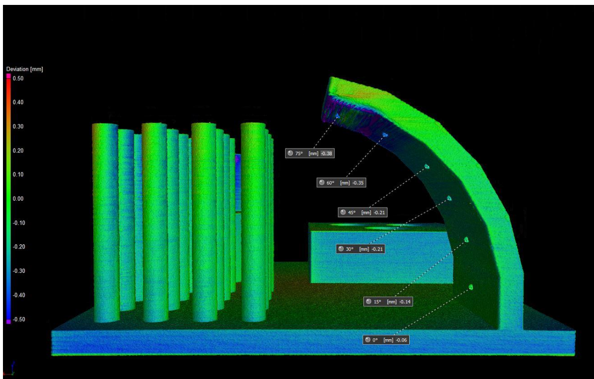
Obr. 4 Převis odchylky Tronxy
