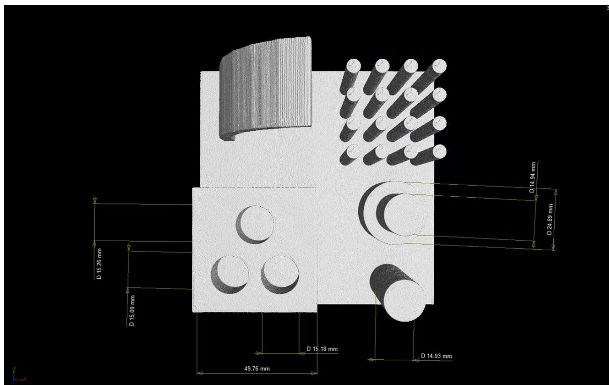
Obr. 6 Rozměry Tronxy
