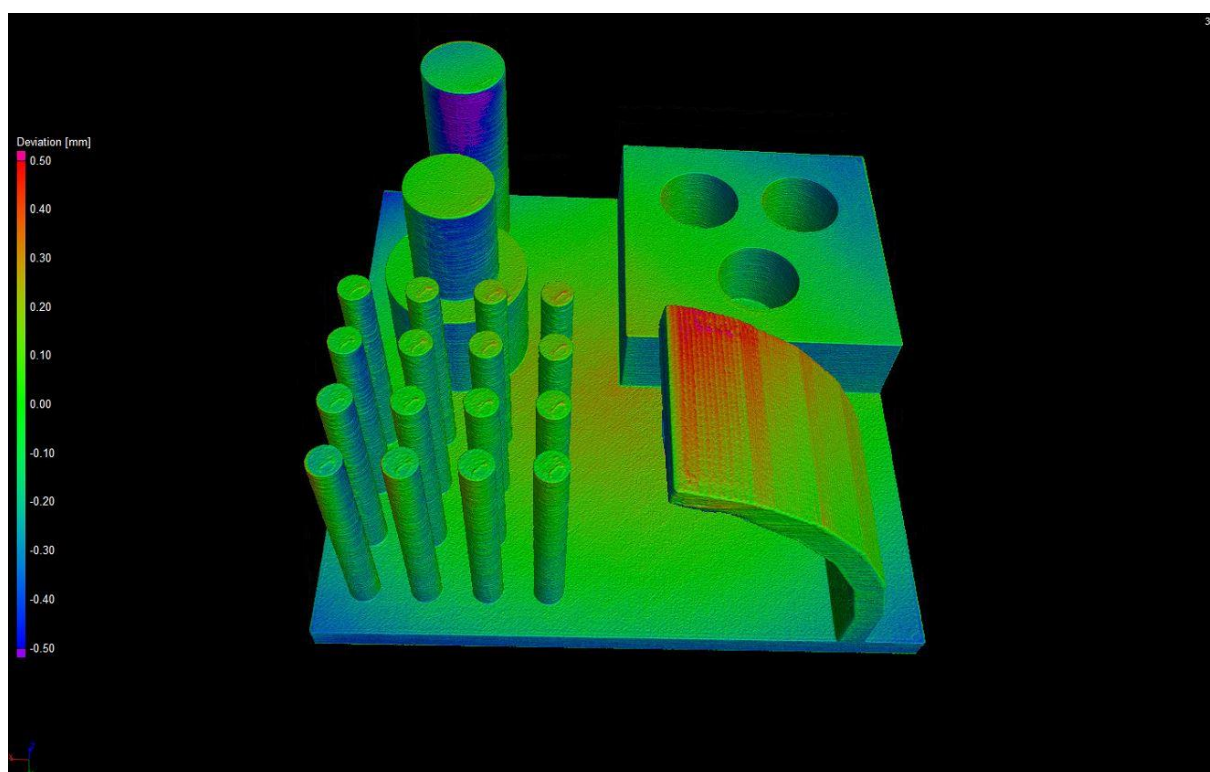
Obr. 2 Barevná mapa zadní Tronxy
