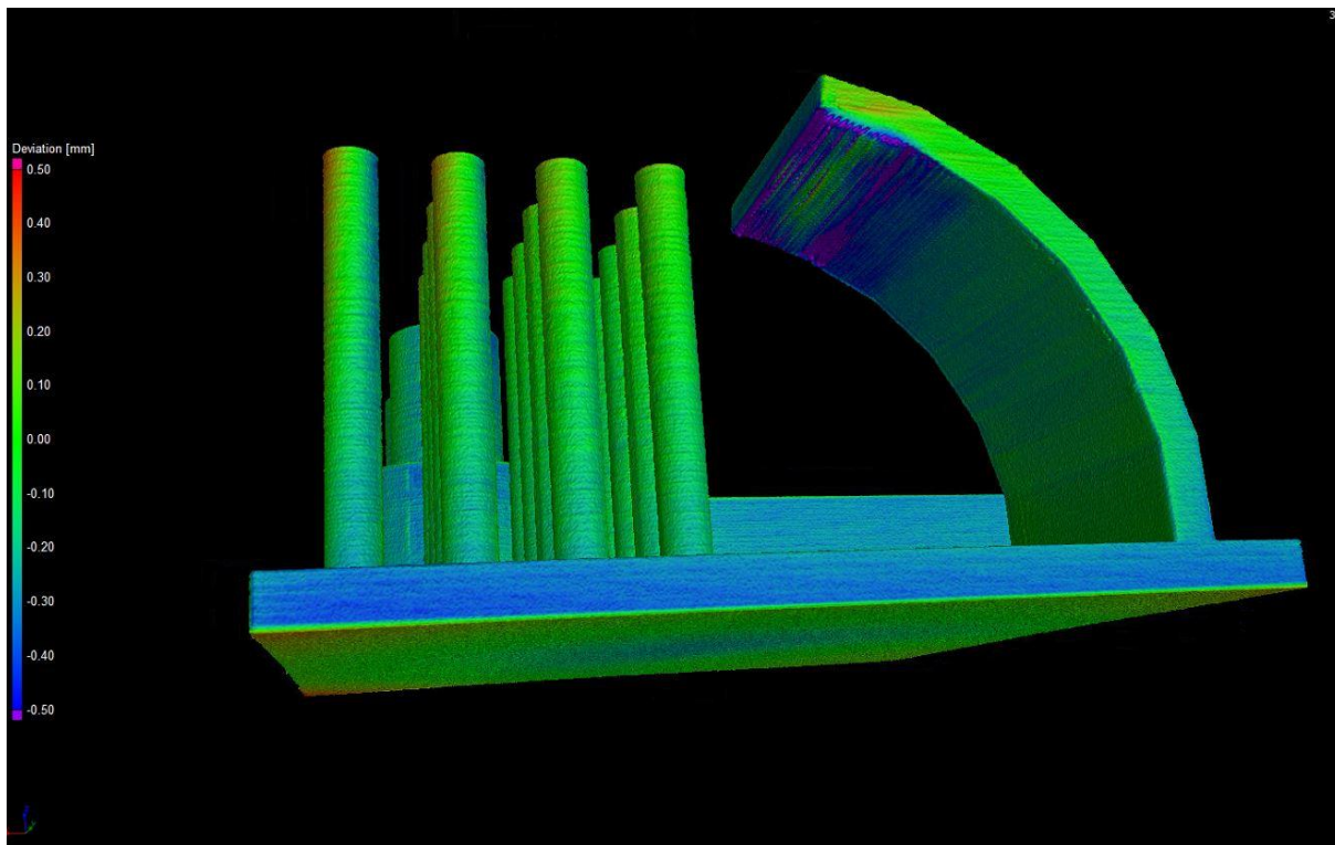
Obr. 3 Převis detail Tronxy
