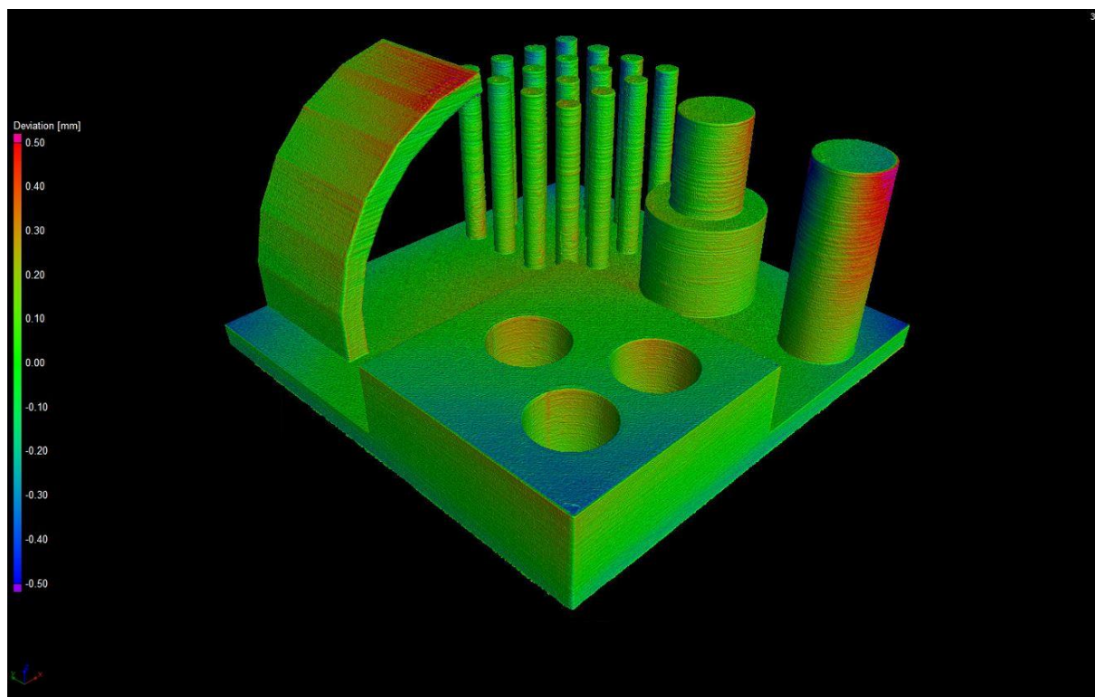
Obr. 1 Barevná mapa Tronxy
