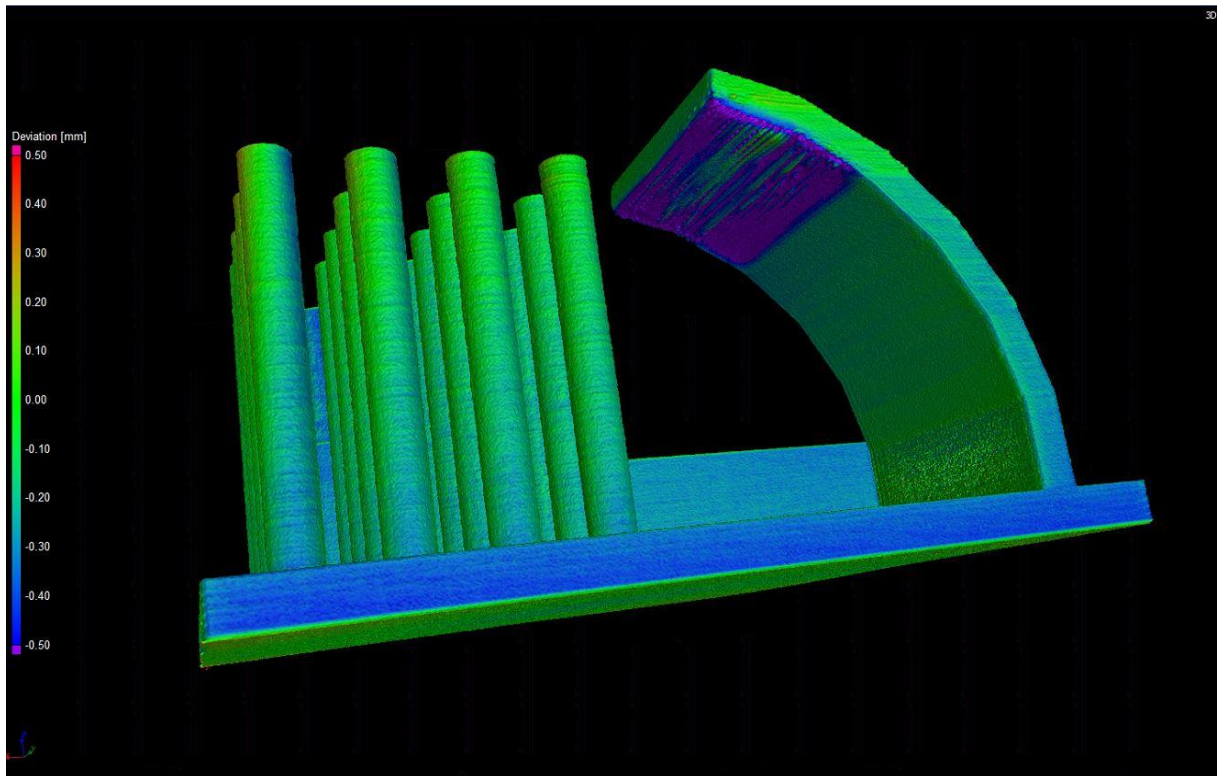
Obr. 3 Převis detail Gembird
