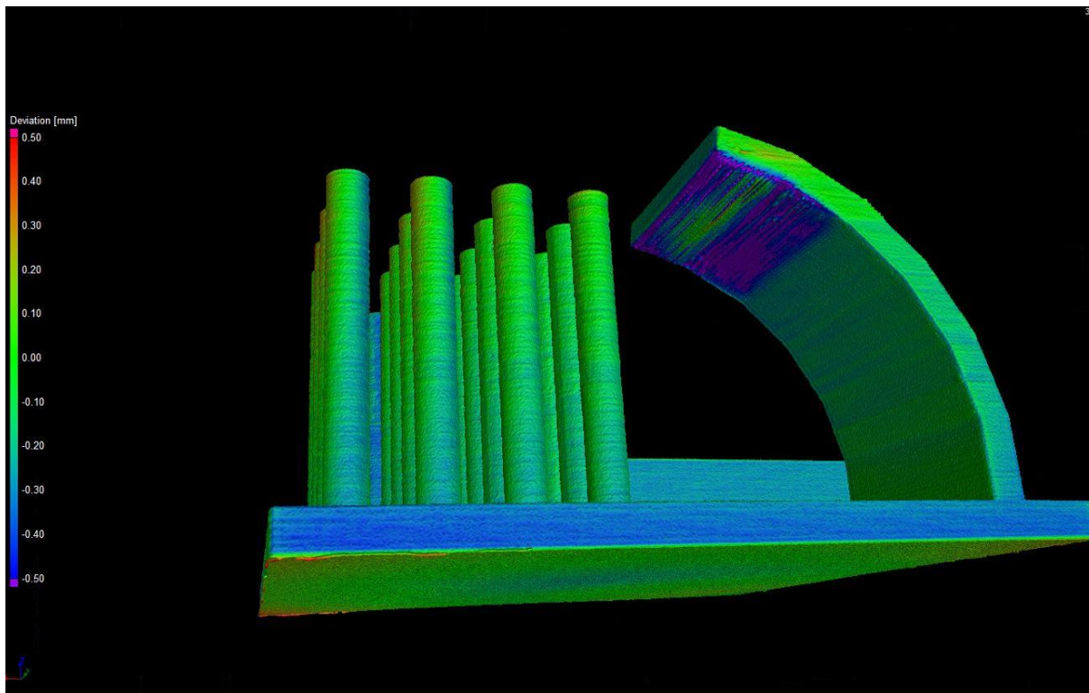
Obr. 3 Převis detail C-Tech
