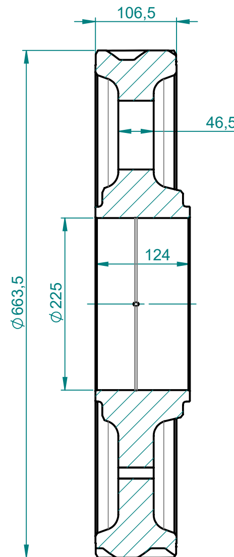
Finální tvar Final shape 1:5
