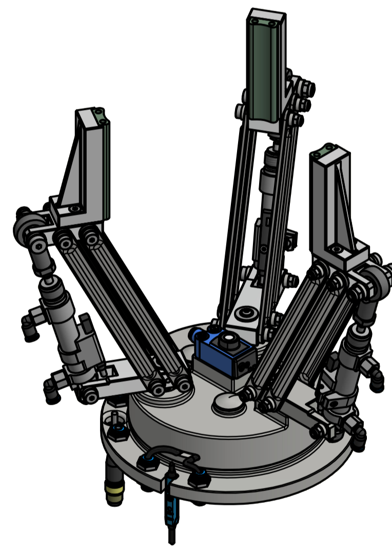
Konfigurace pro uchopení rotačního dílce
