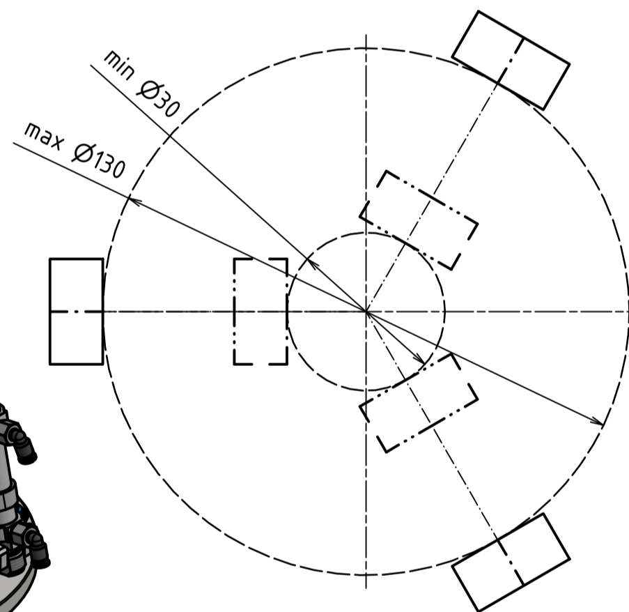
Konfigurace pro uchopení rotačního dílce
