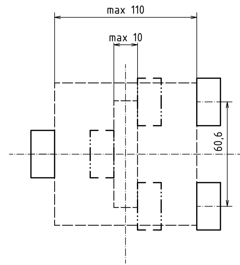
Konfigurace pro uchopení prizmatického dílce
