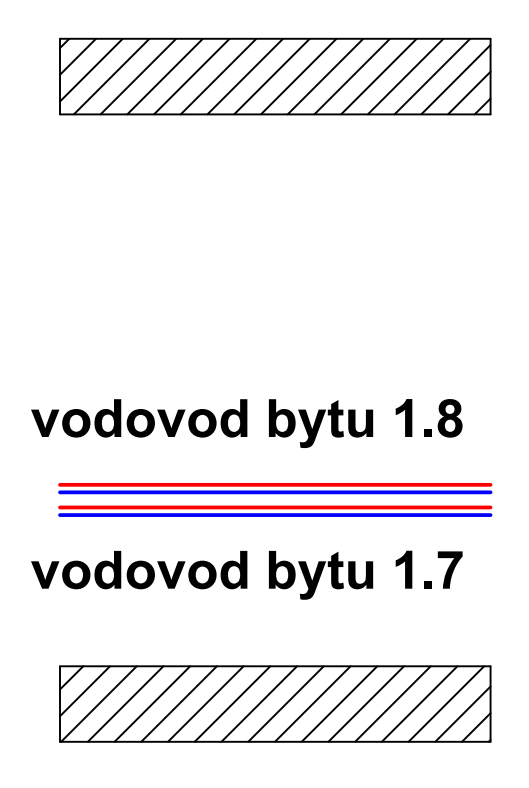
DETAIL 3 vedení vodovodu ve stěně
