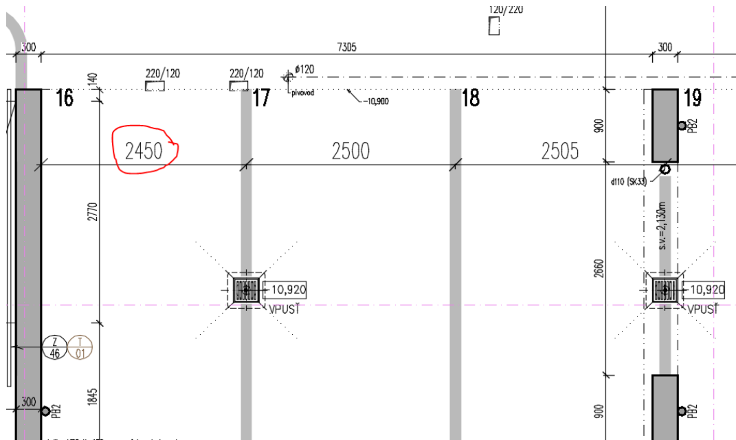
Obrázek 1 - Výřez půdorysu 3PP
