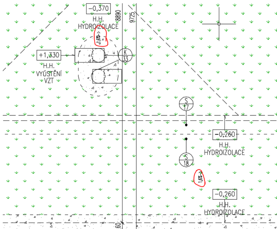
Obrázek 3 - Výřez půdorysu 1.NP
