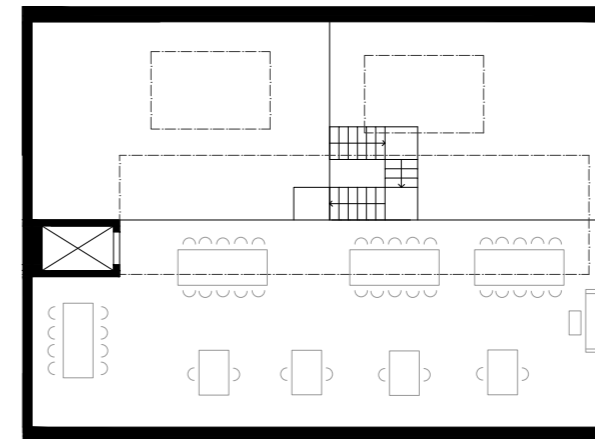
PŮDORYS 3.NP
