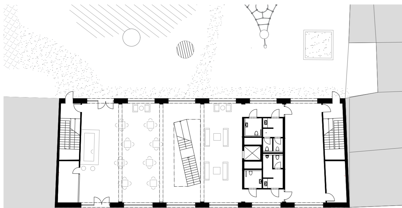
PŮDORYS 1.NP
