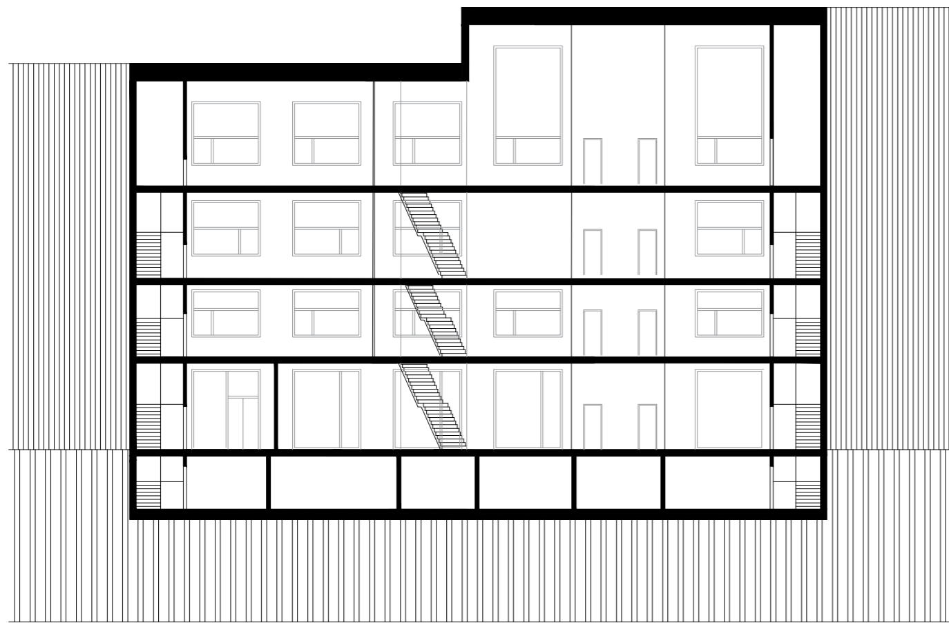
ŘEZ PODÉLNÝ
