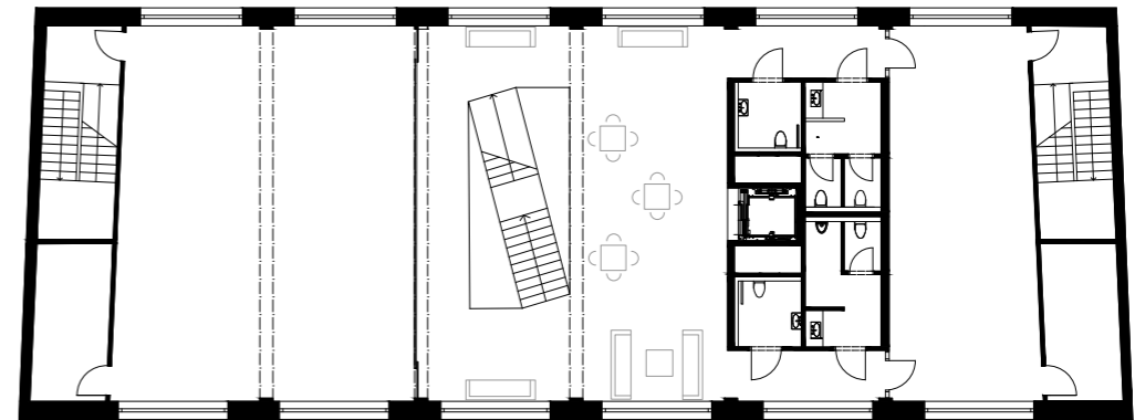
PŮDORYS 2.NP
