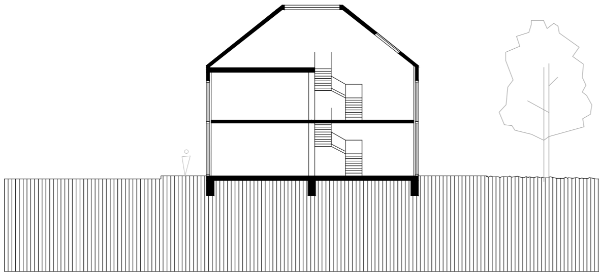
ŘEZ PŘÍČNÝ
