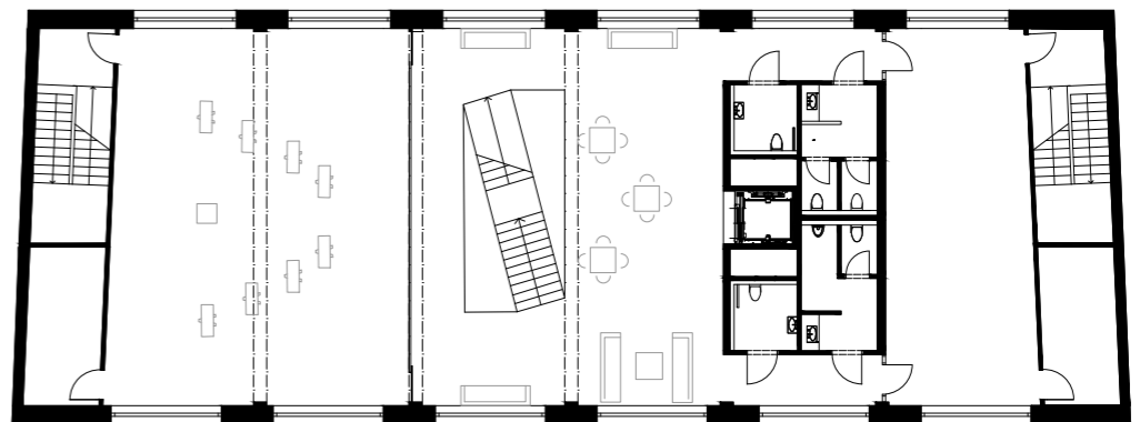
PŮDORYS 3.NP
