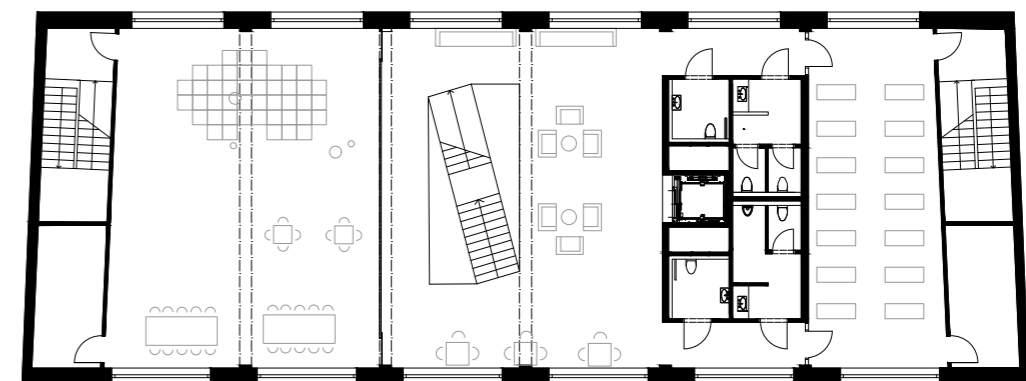
PŮDORYS .NP
