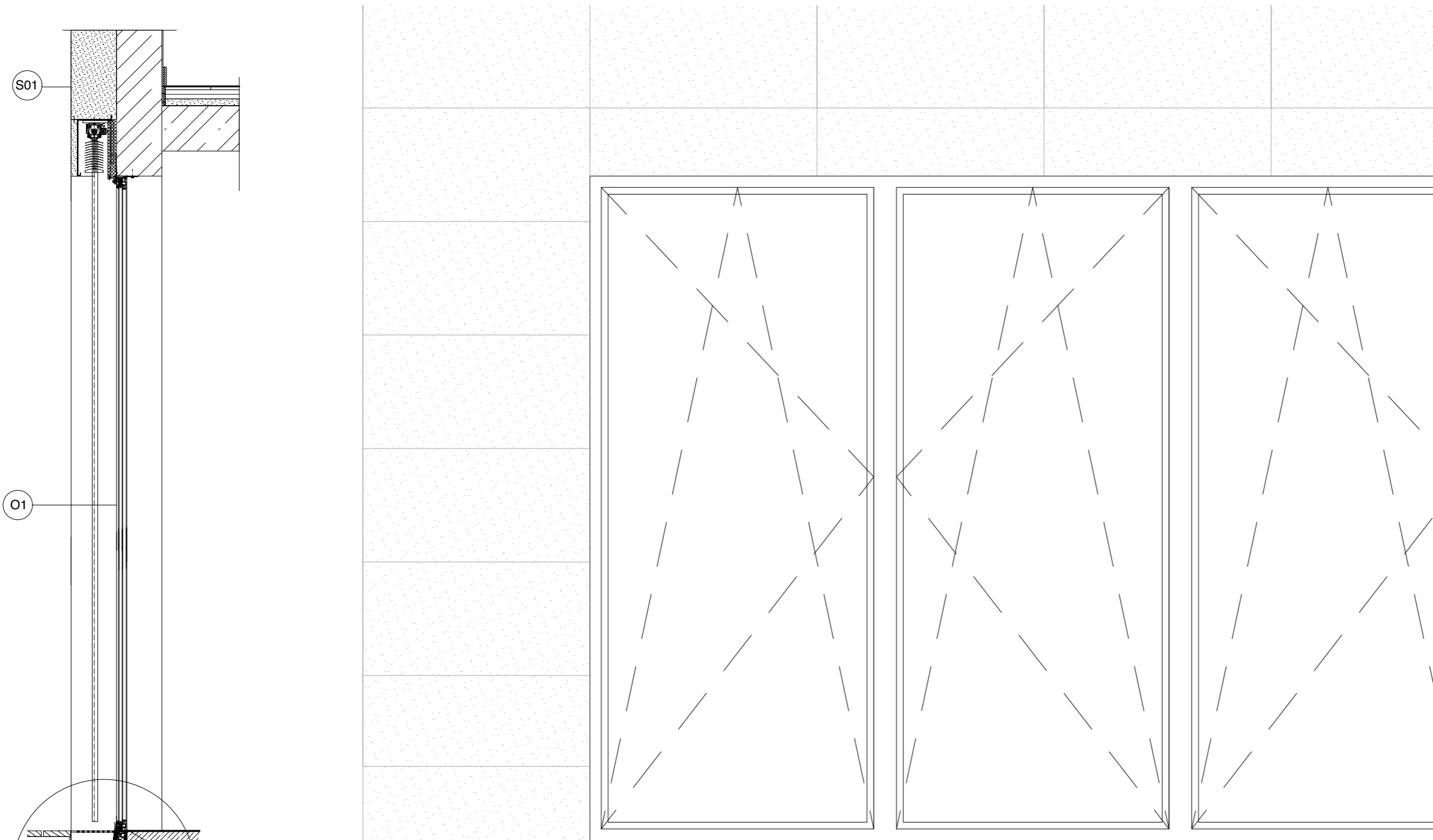
SYSTÉMOVÝ DETAIL KOTVENÍ FRANCOUZSKÝCH OKEN SCHUCO
