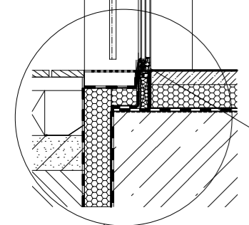
SYSTÉMOVÝ DETAIL KOTVENÍ FRANCOUZSKÝCH OKEN SCHUCO
