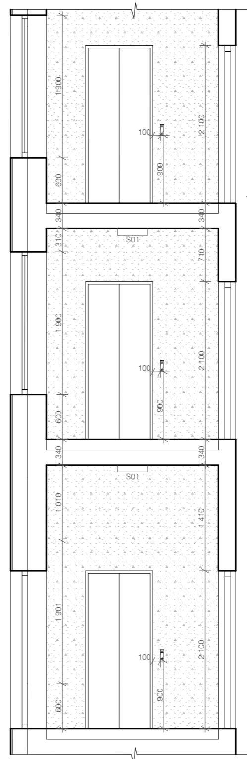
Řez BB'
