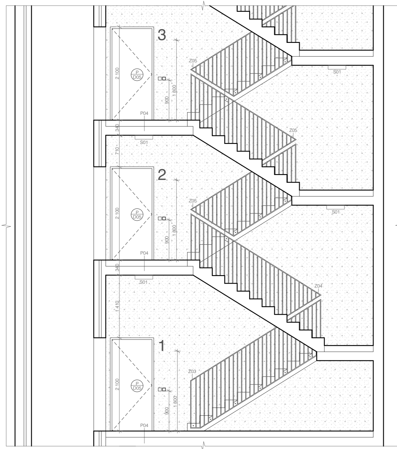
Řez AA'
