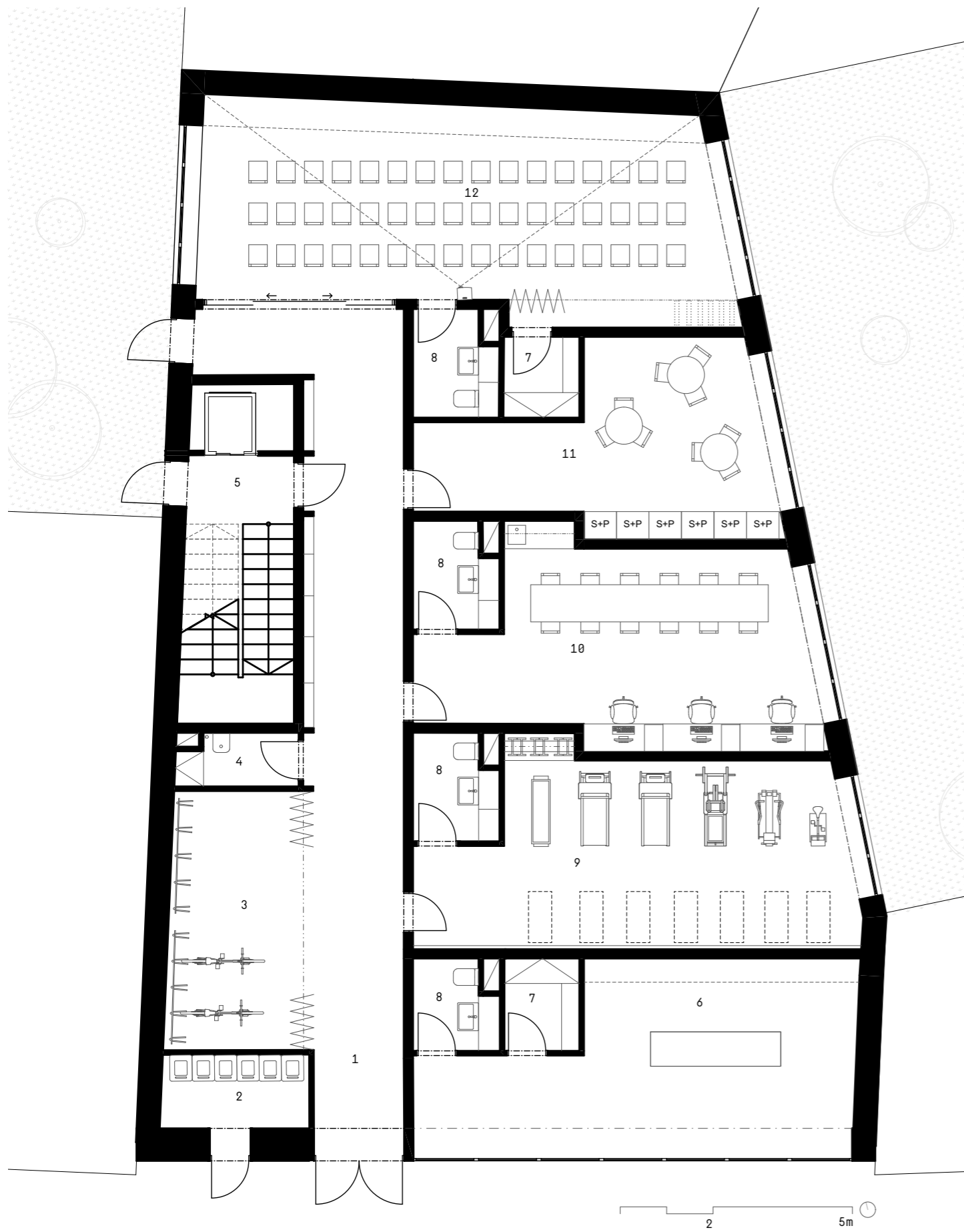
Půdorys 1.NP
